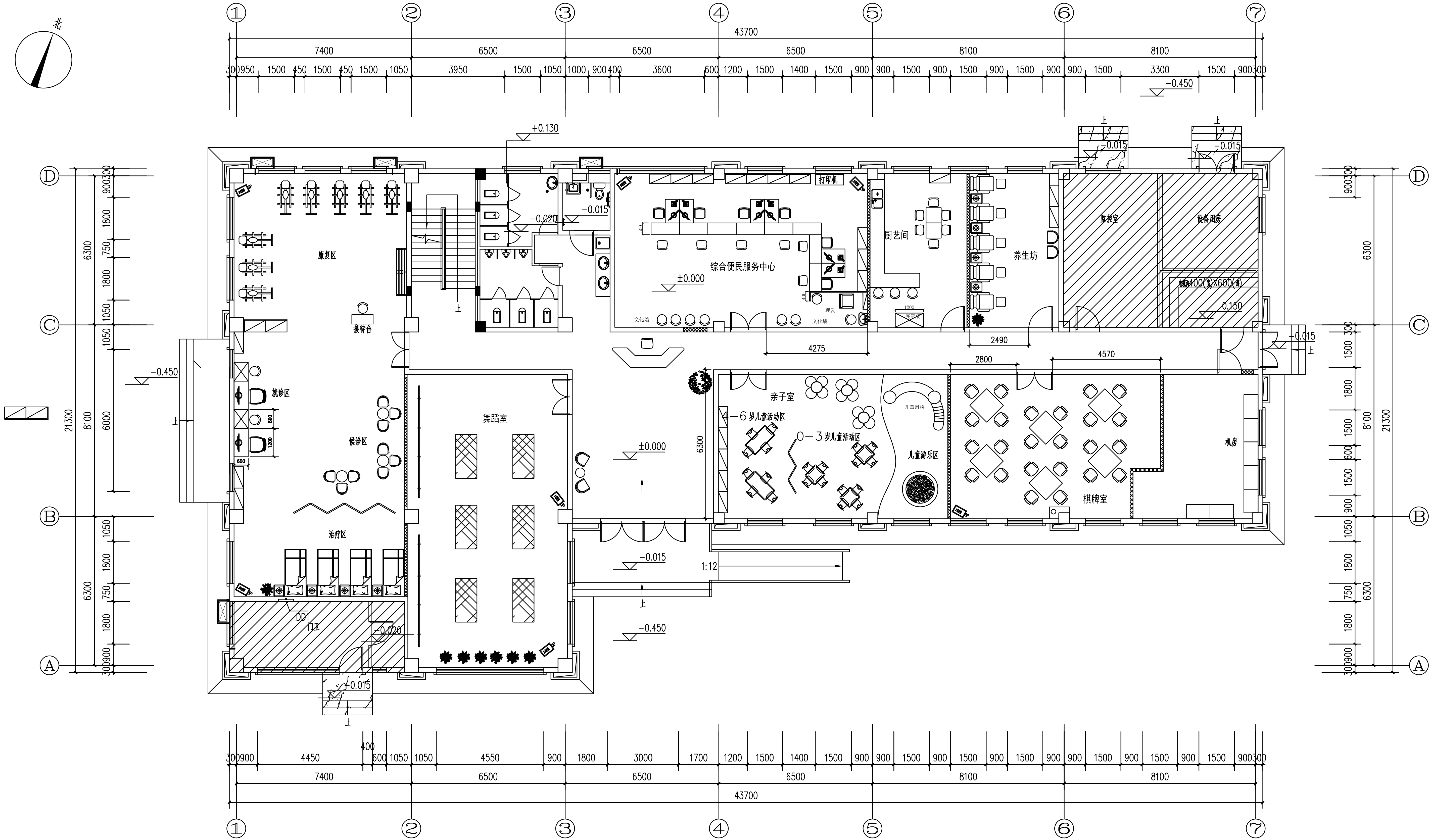
一层平面图 1:100
