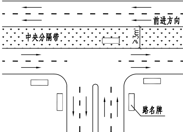
丁字路 E2型
