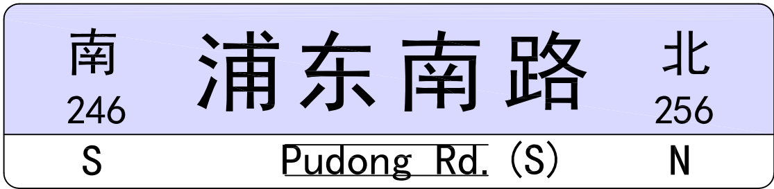
A型4字体版面布置图 1:10
