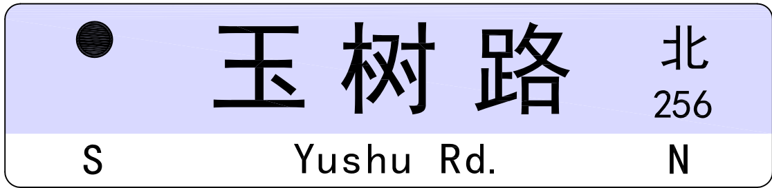
A型3字体断头版面布置图 1:10
