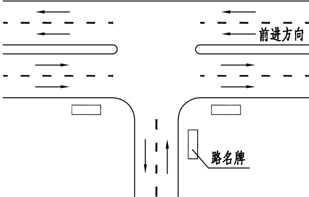
丁字路 D型
