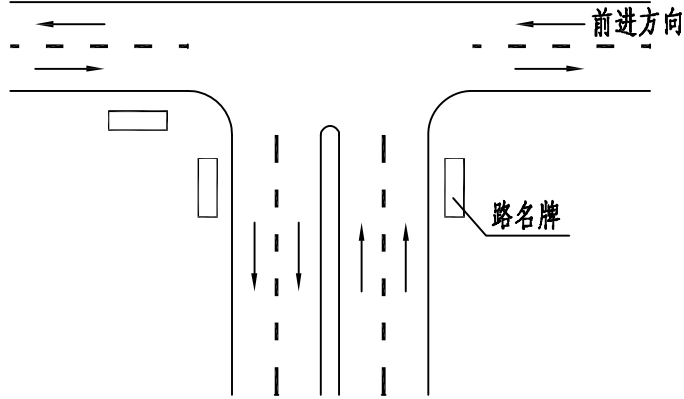
丁字路 C型
