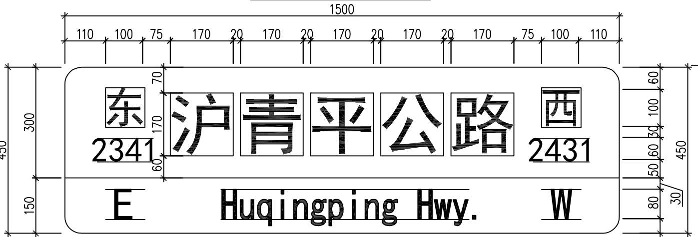
B型3字体端头版面布置图 1:10
