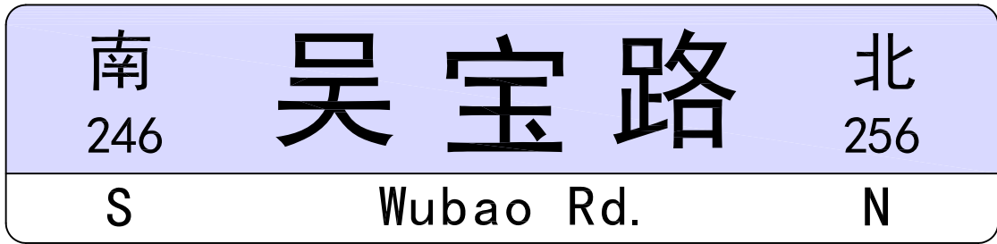
A型3字体版面布置图 1:10
