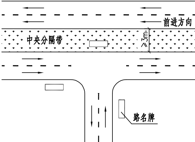
丁字路 E1型
