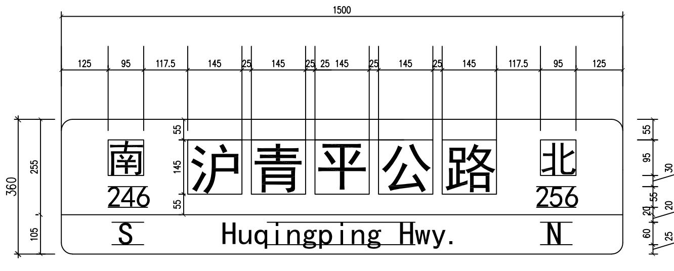
A型3字体断头版面布置图 1:10
