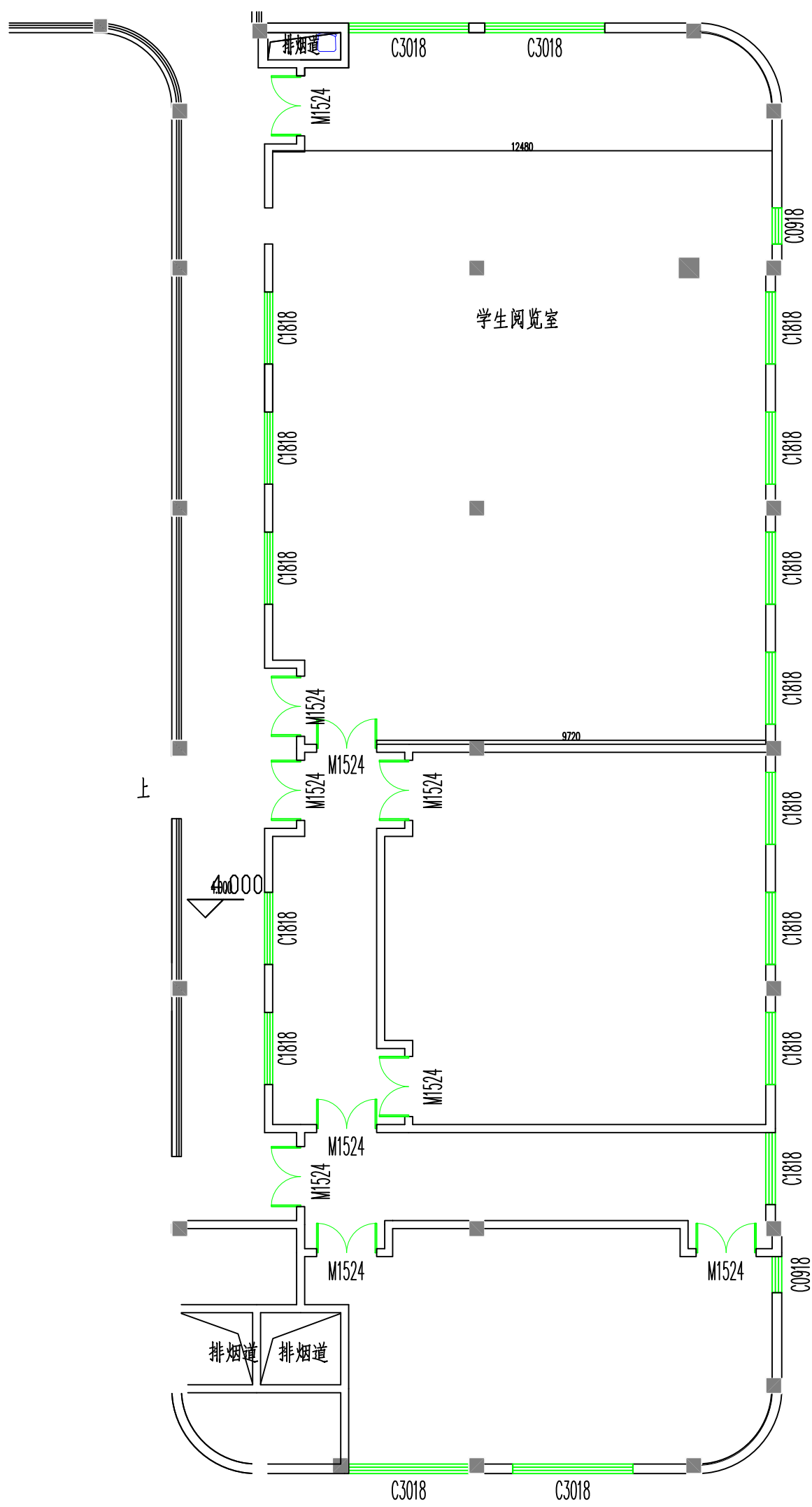
二号楼二层图书馆平面图
