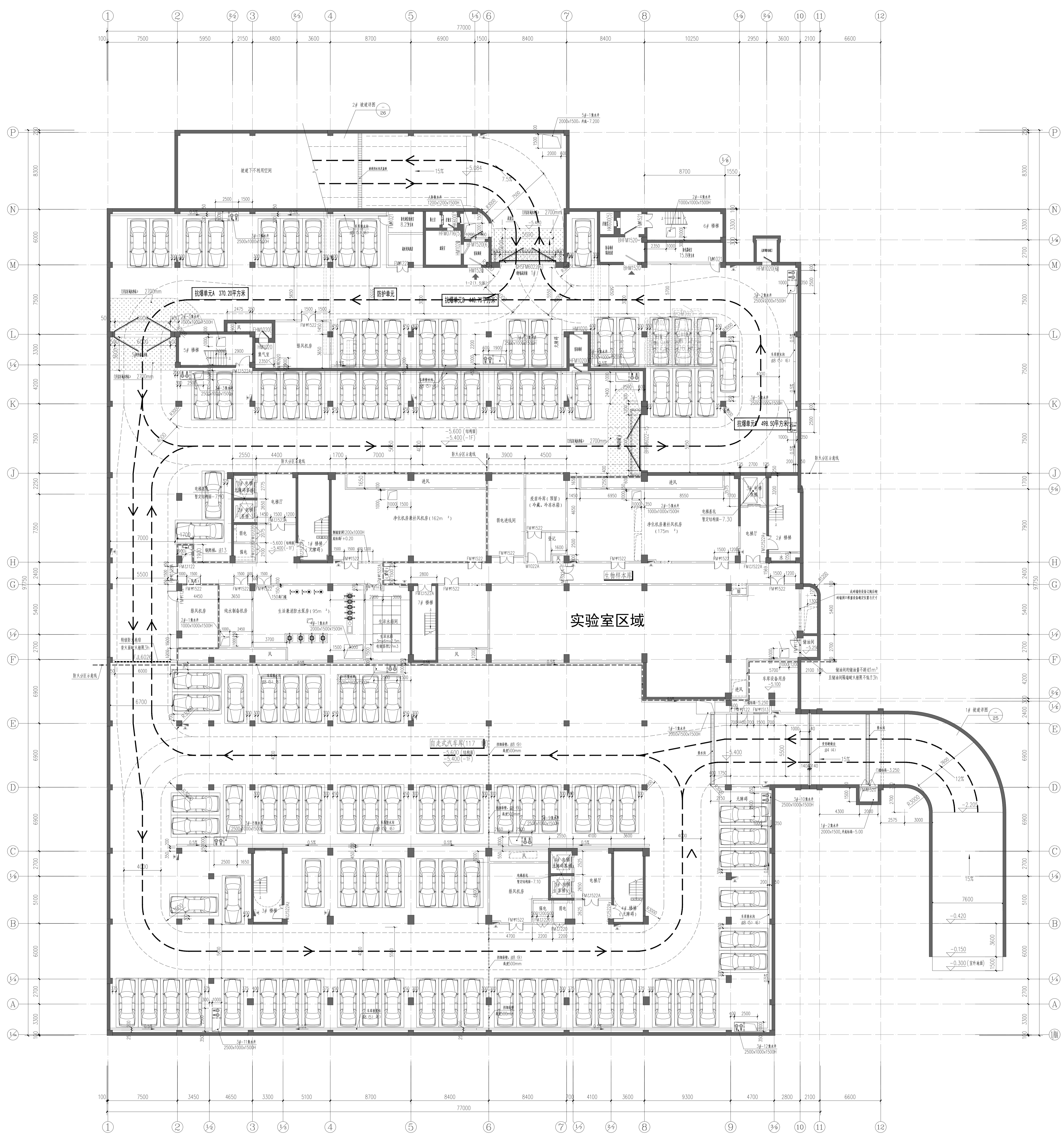
地下一层平面图(平时) 1:150
