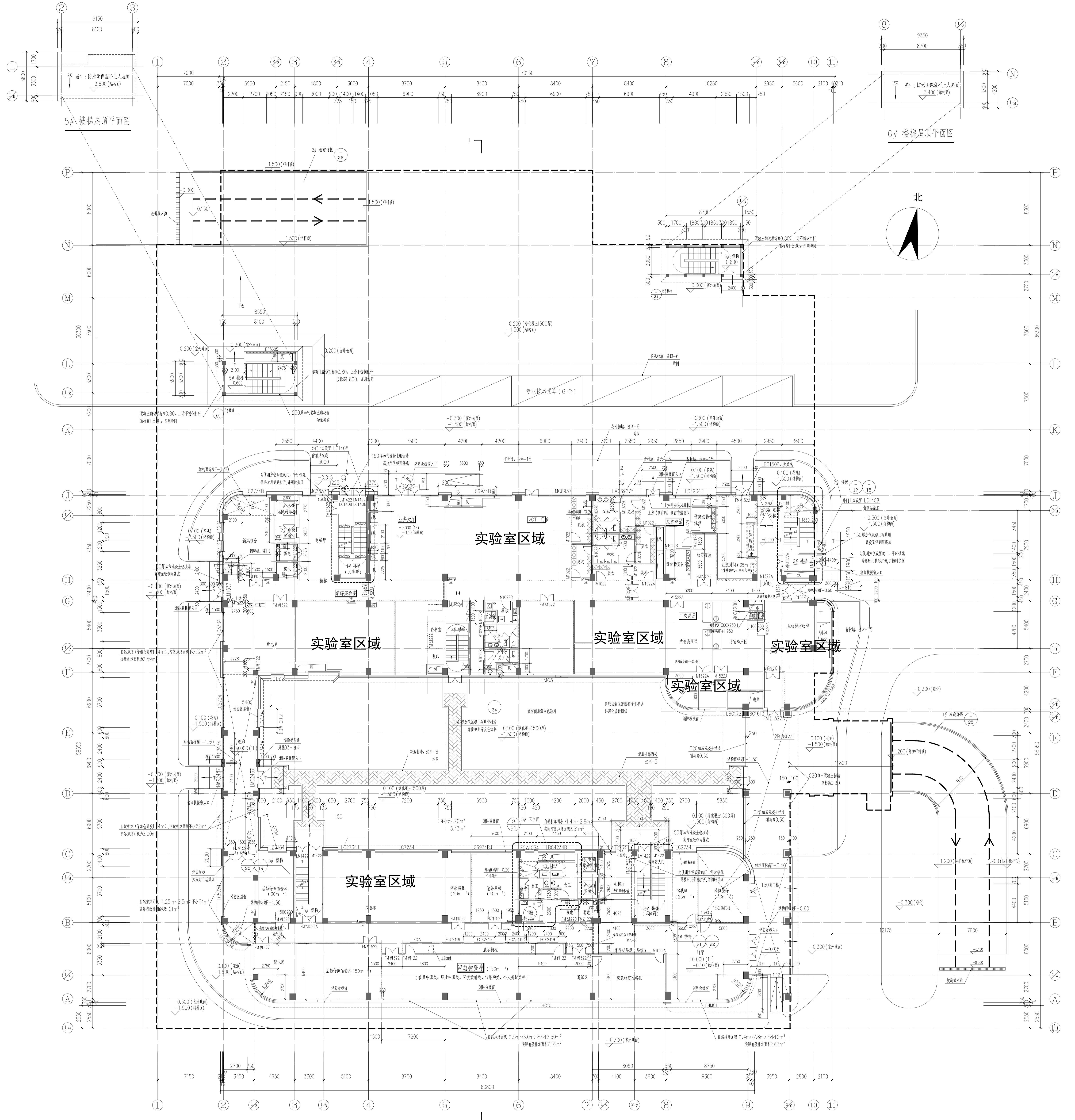
一层平面图 1:150
