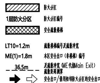
防火分区图例
