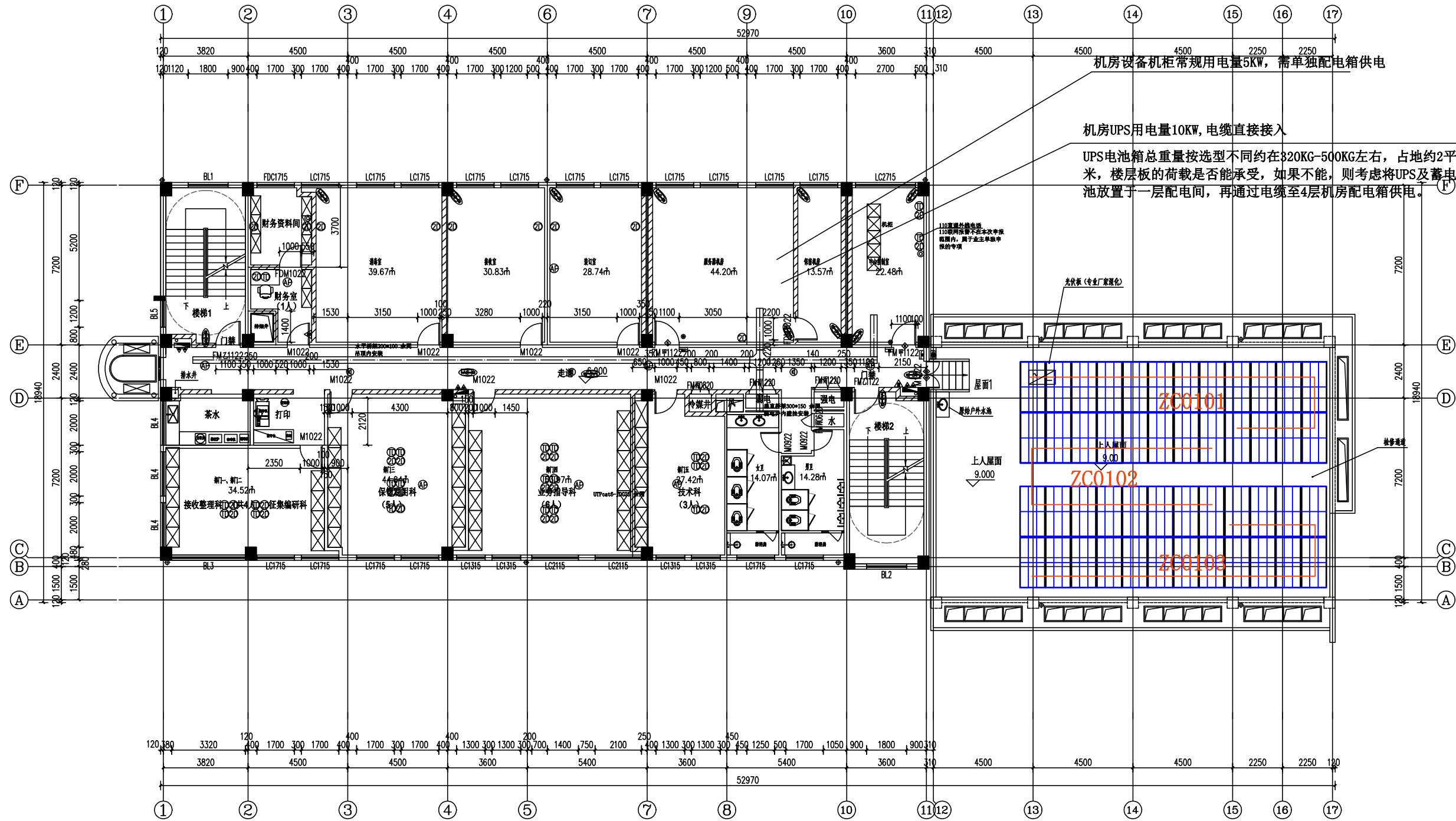
四层平面图 1:100
