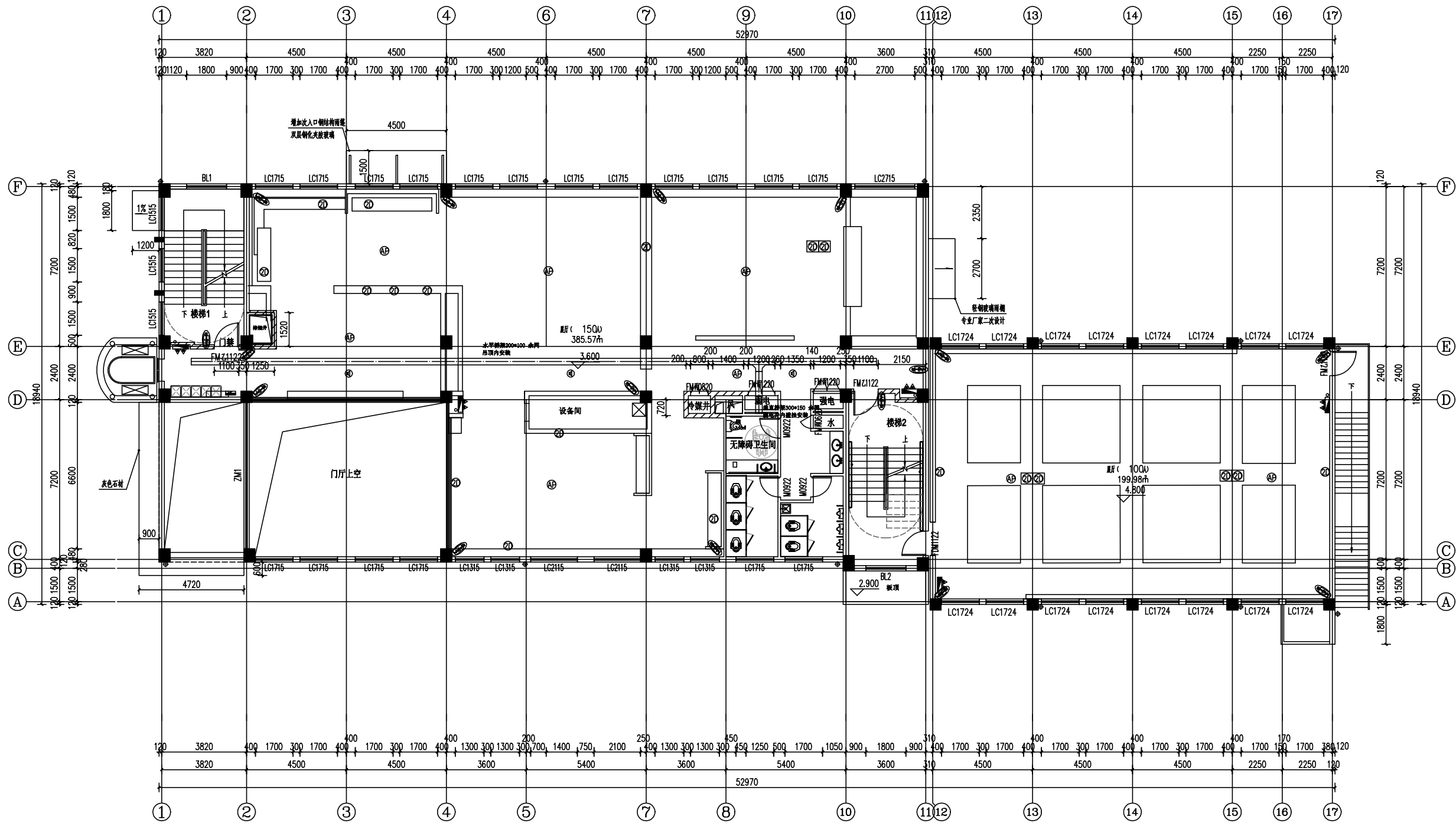
二层平面图 1:100
