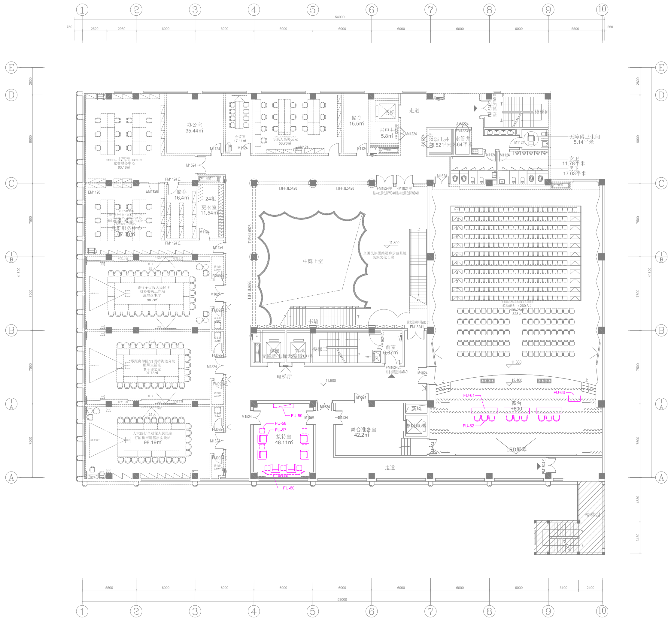
四层平面图
