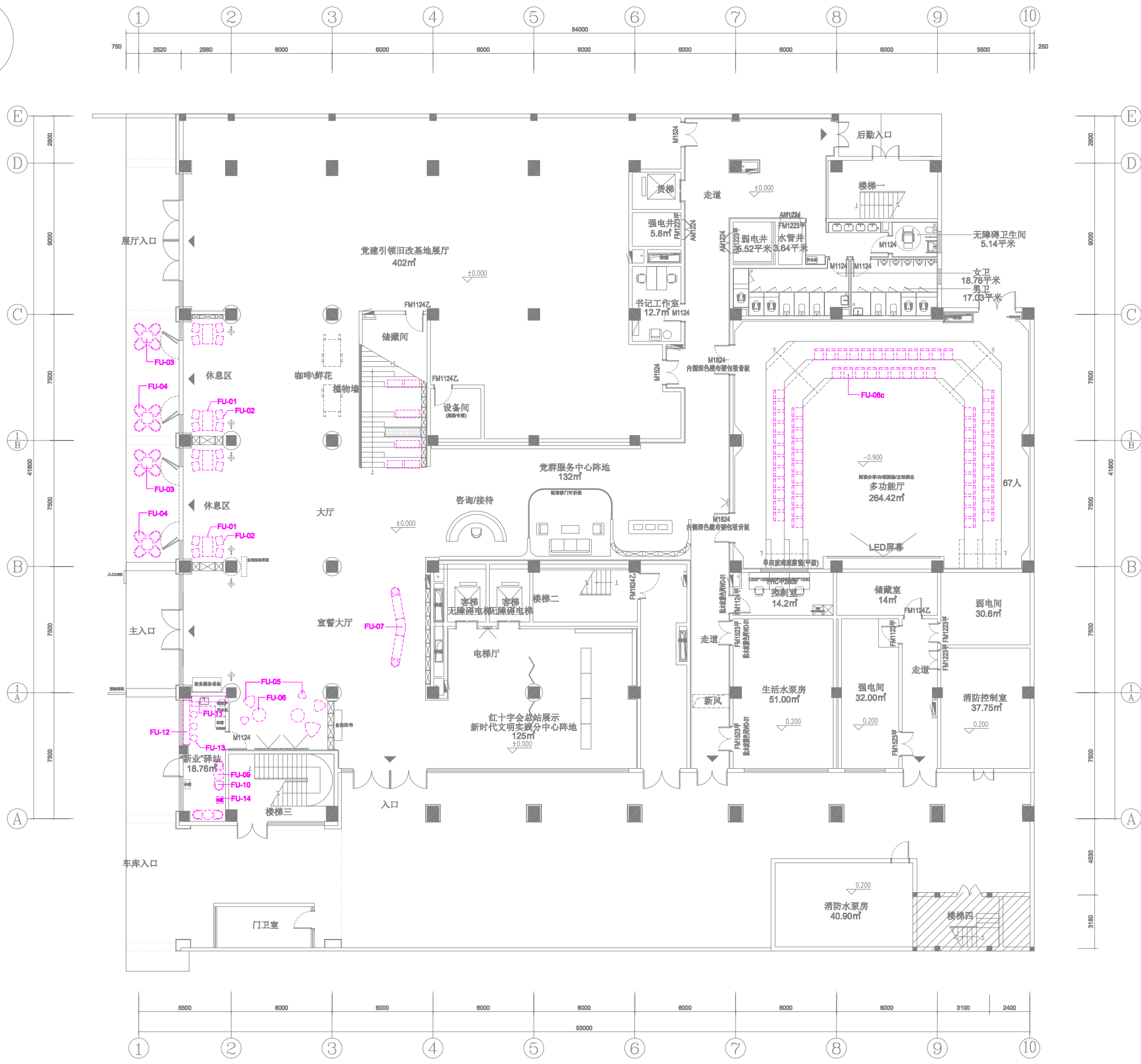
一层平面图
