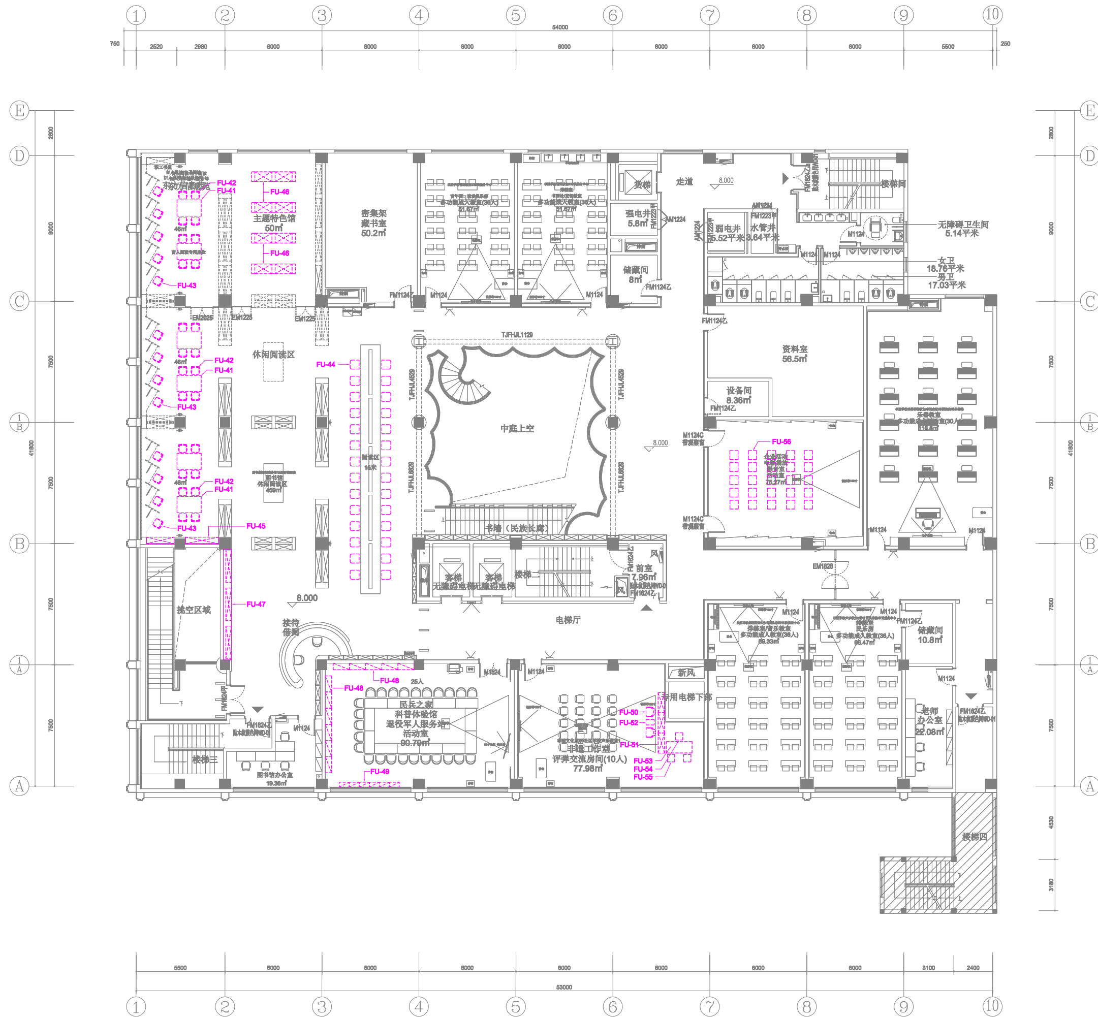
三层平面图
