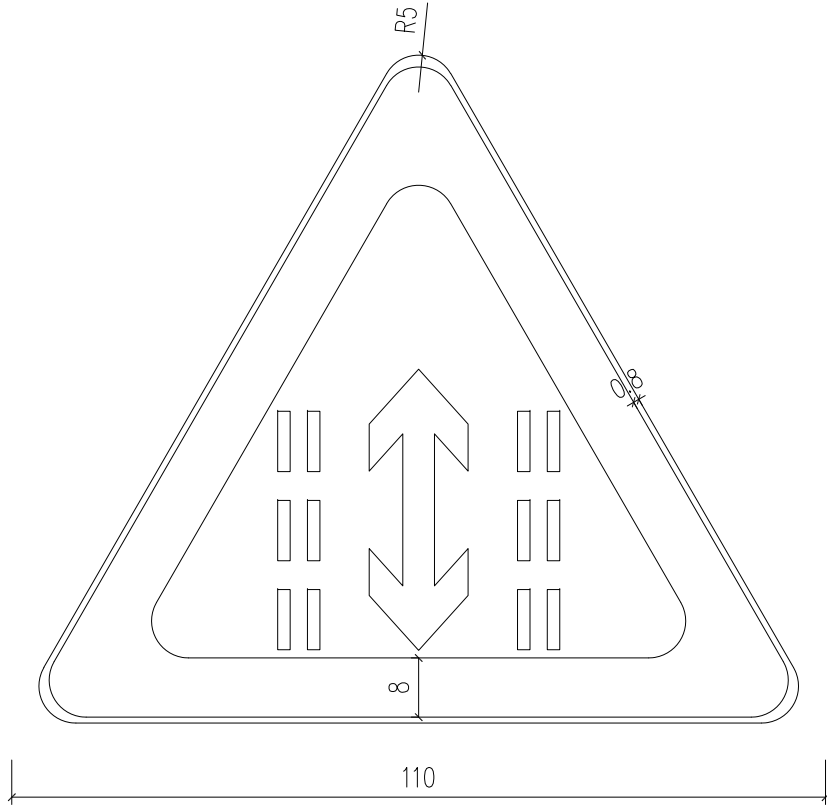
潮汐车道标志(一) 1:10
