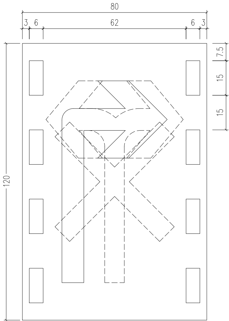
LED可变标志(四) 1:10
