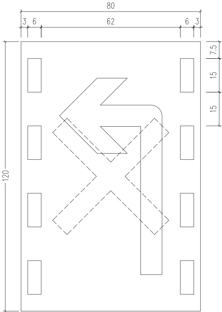
LED可变标志(三) 1:10
