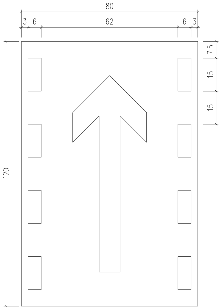
LED可变标志(一) 1:10
