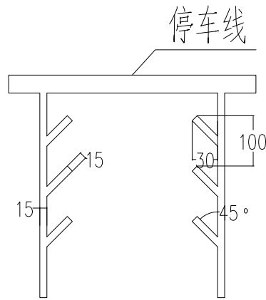
可变导向车道标线 单位：cm 1:50
