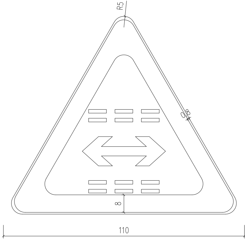
潮汐车道标志(二) 1:10
