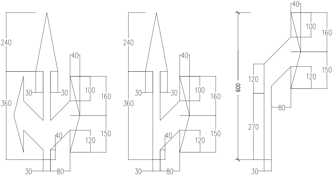
箭头大样图 单位：cm 1:50
