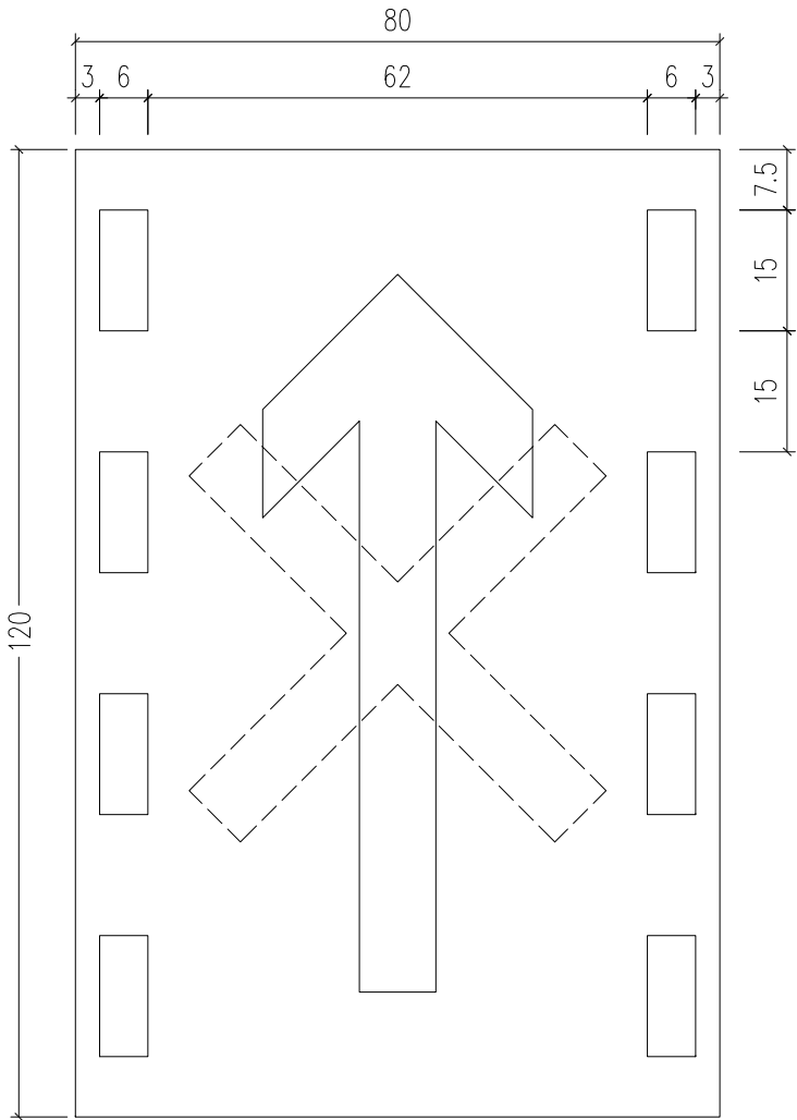
LED可变标志(二) 1:10
