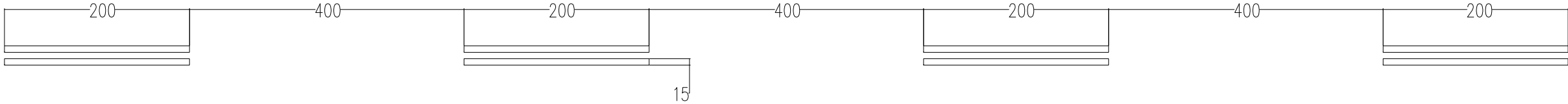
潮汐车道标线大样图 单位：cm 1:50
