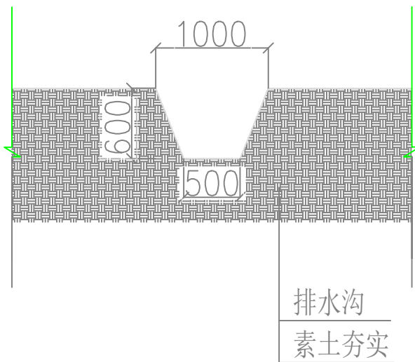
4 一级排水沟-作法详图
