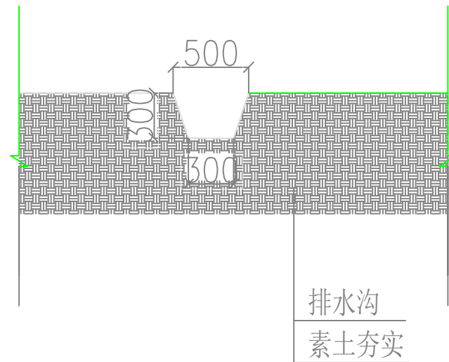
5 二级排水沟-作法详图
