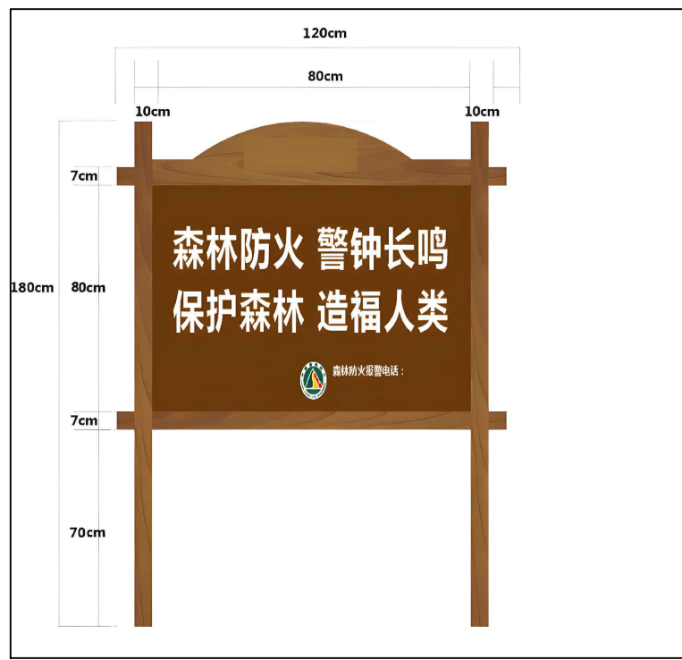
2 标识牌-森林防火示意图
