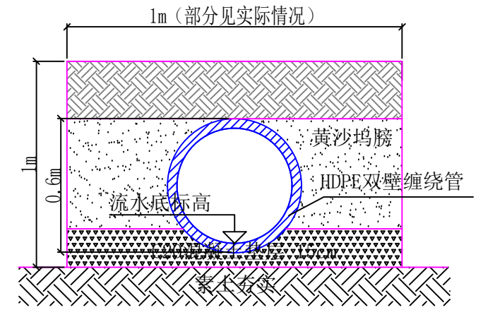
3 涵管剖面详图
