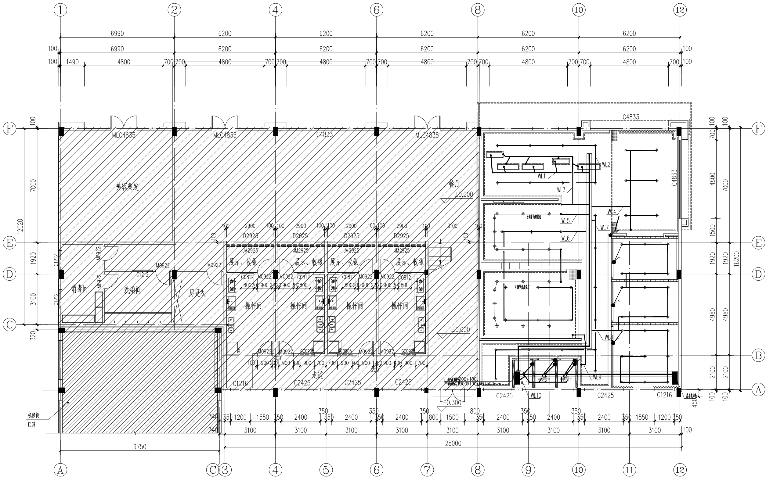
一层天花造型布线图 1:100
