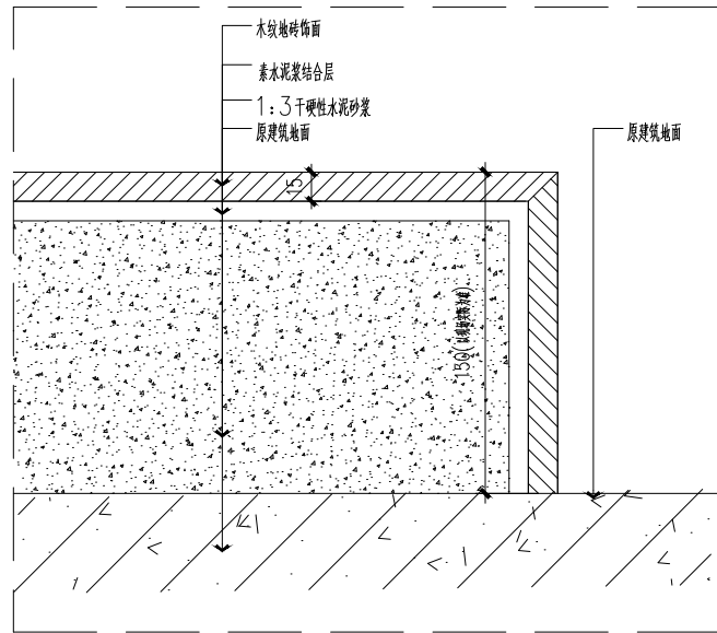
01大样图 比例1:3
