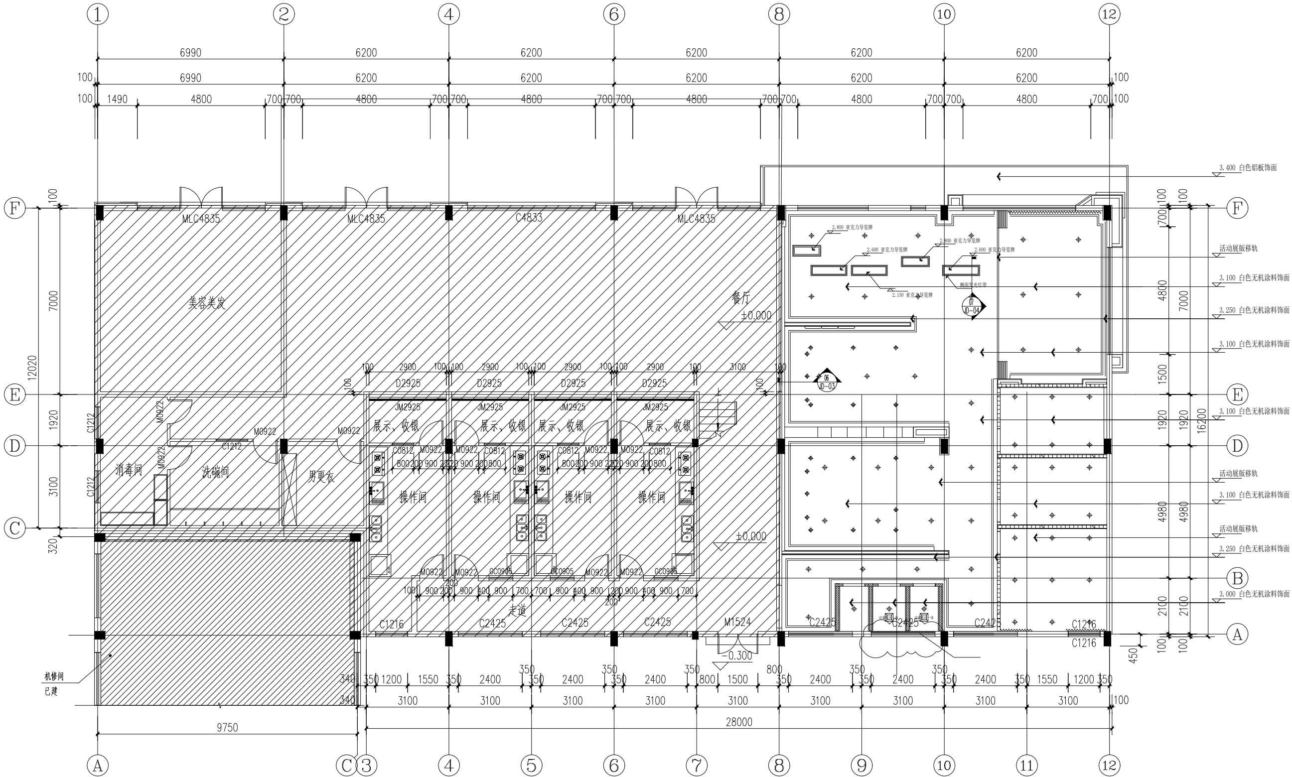
一层天花造型布置图 1:100
