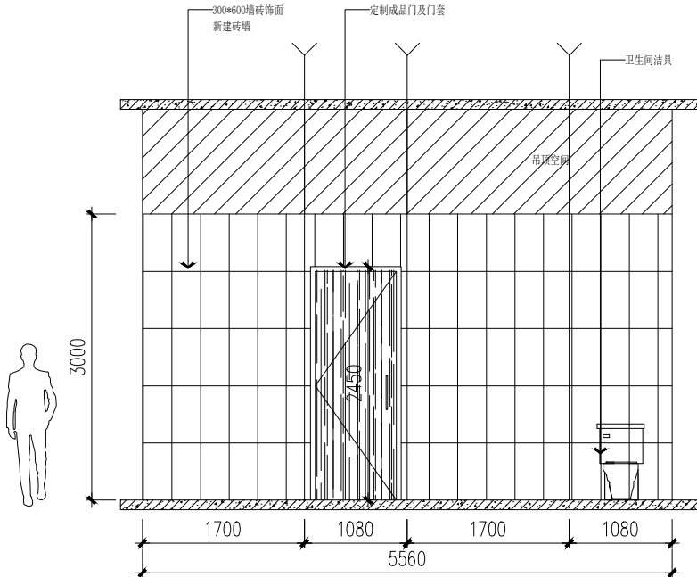
26立面图 比例1:40
