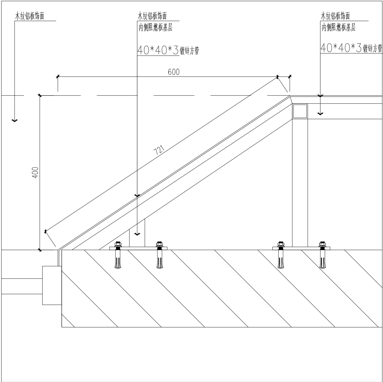
11大样图 比例1:4
