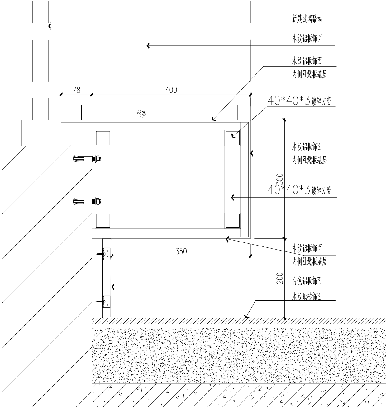
10大样图 比例1:4
