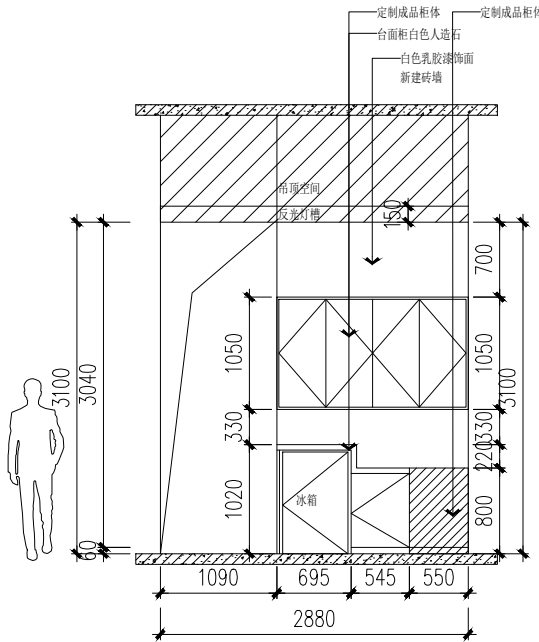
24立面图 比例1:40
