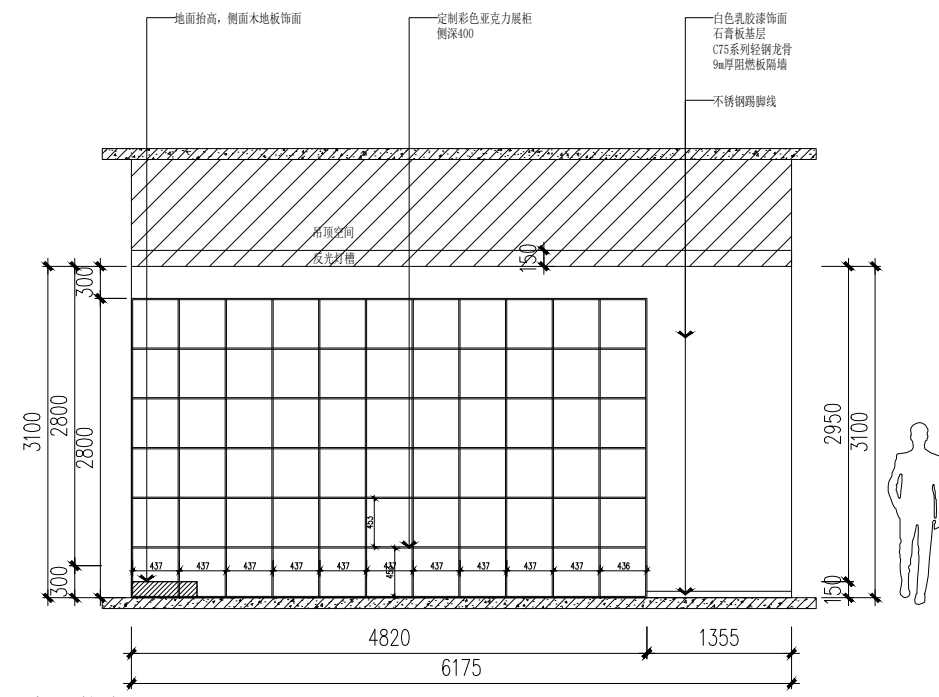
14立面图 比例1:40
