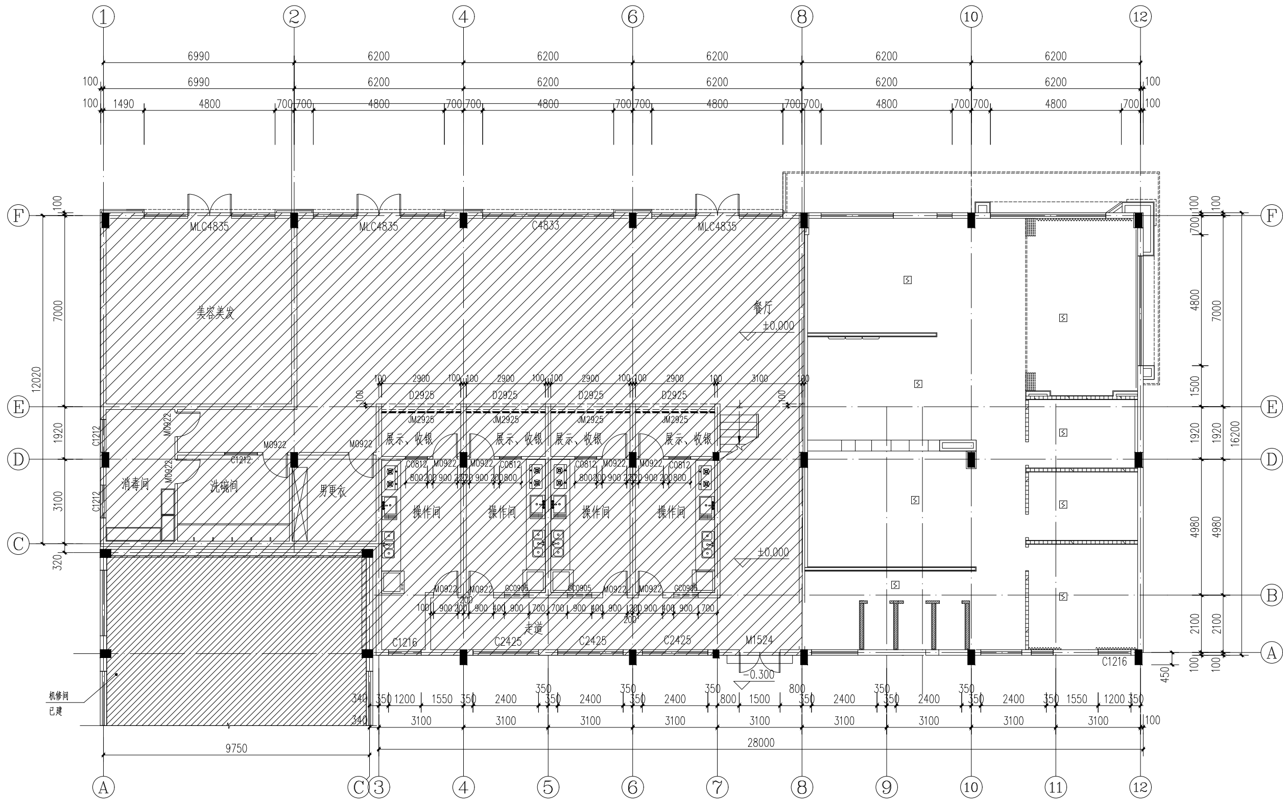
一层烟感点位图 1:100
