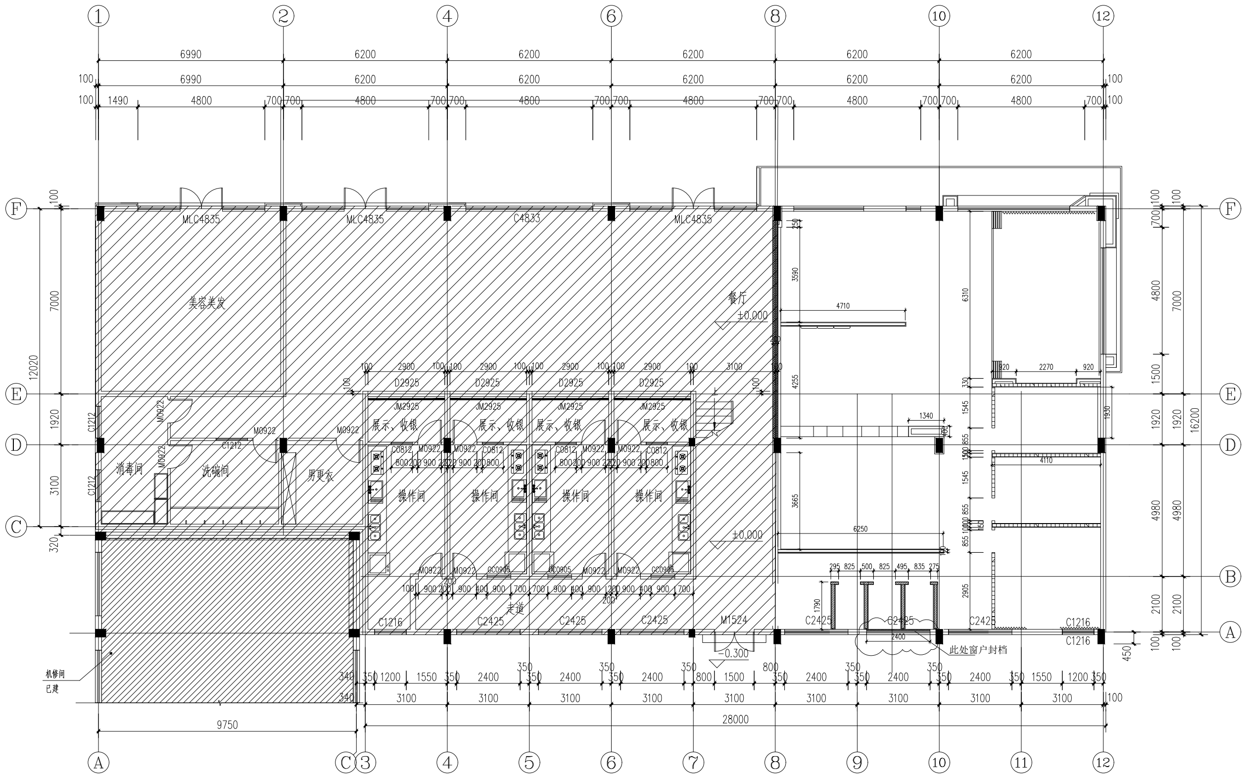
一层新建隔墙定位图 1:100
