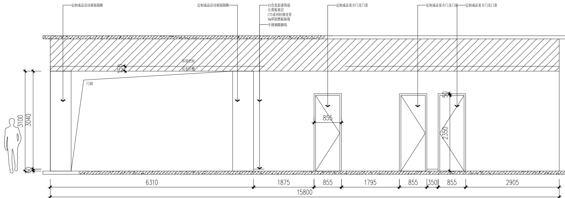
08立面图 比例1:40
