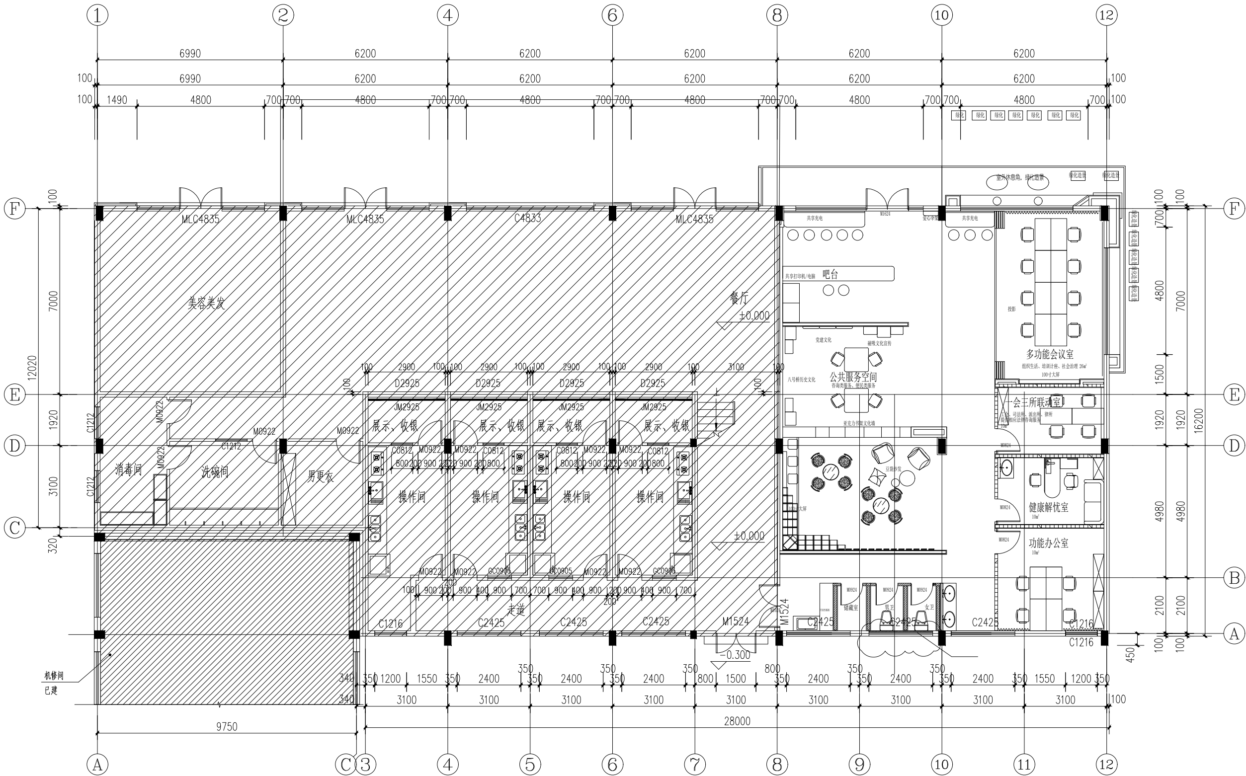
一层平面布置图 1:100
