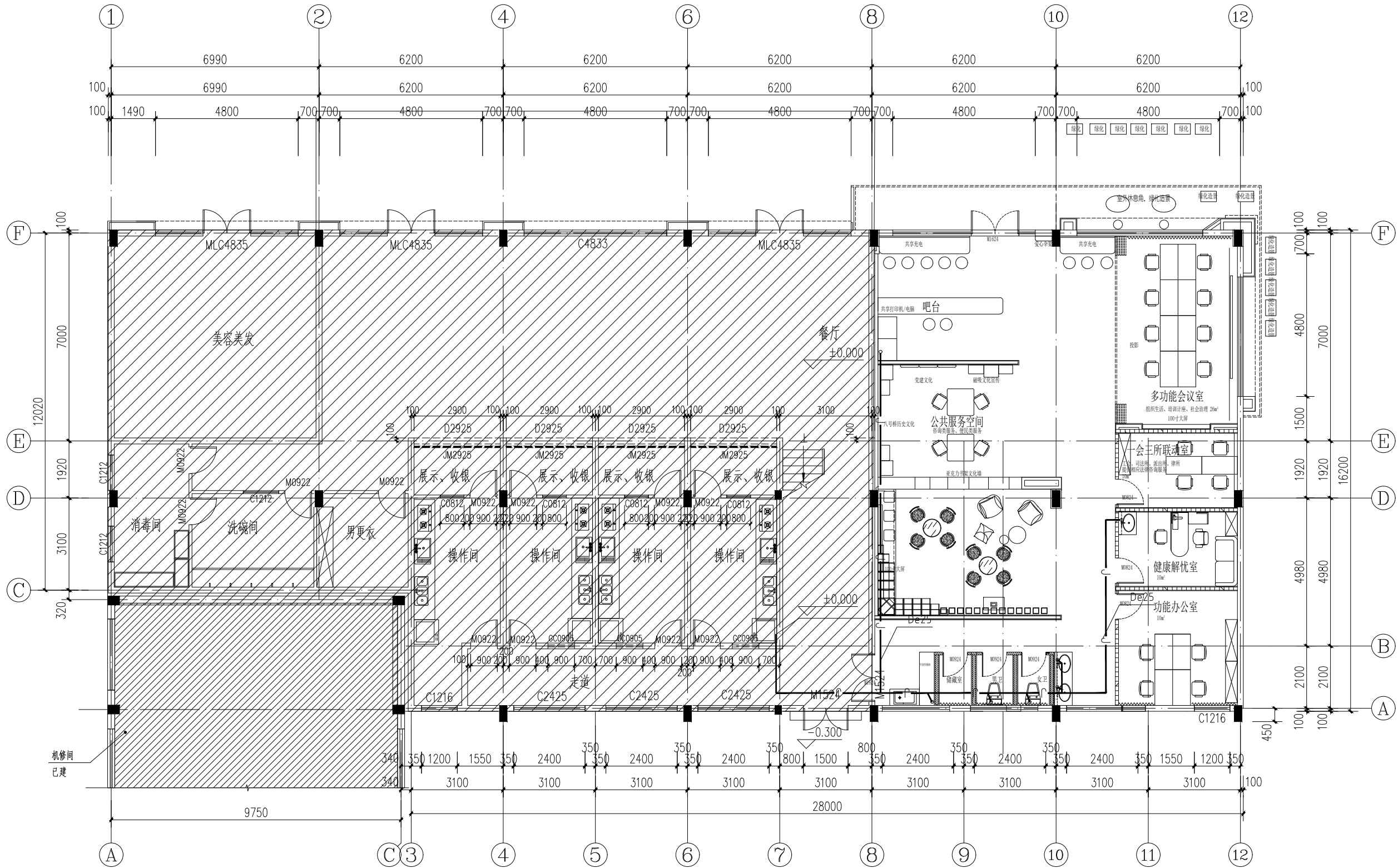
一层给水平面图 1:100
