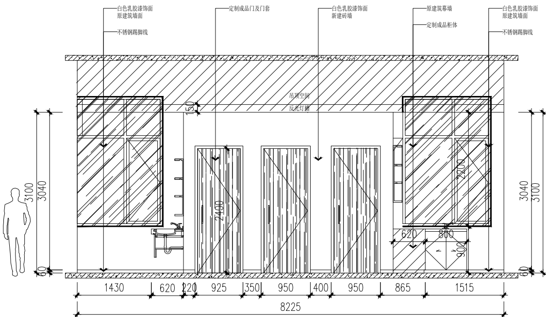
22立面图 比例1:40
