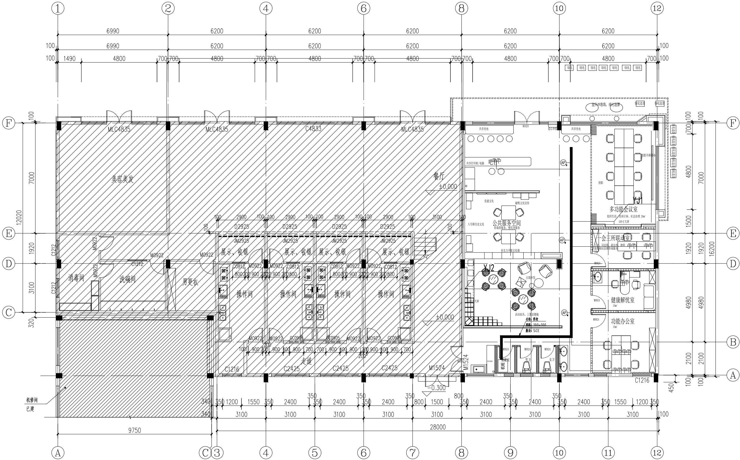
一层弱电布线平面图 1:100
