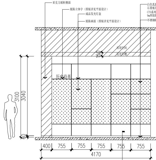
12立面图 比例1:40
