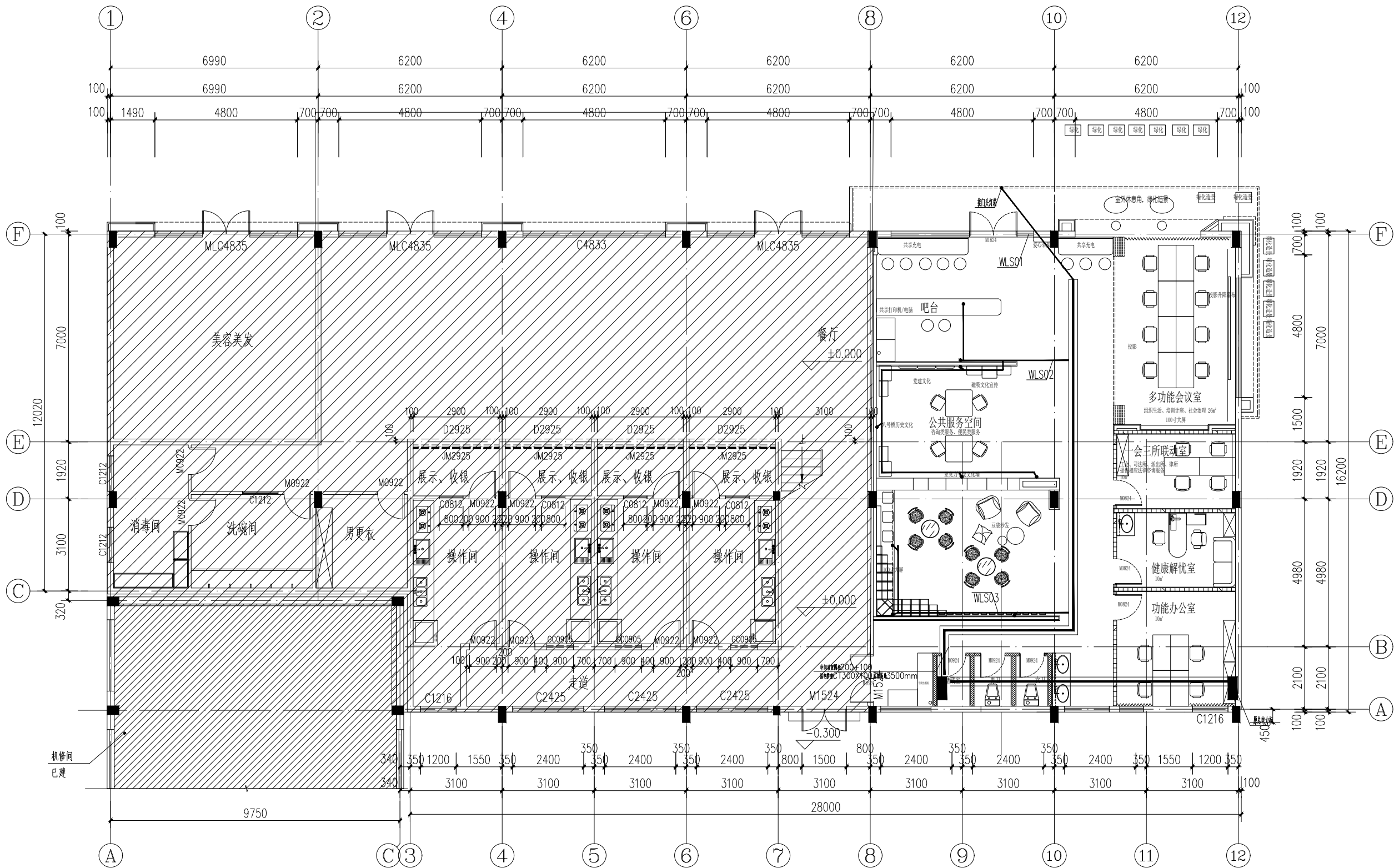
一层立面照明布线图 1:100
