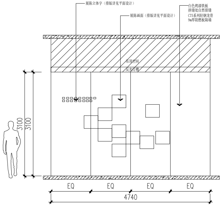
11立面图 比例1:40
