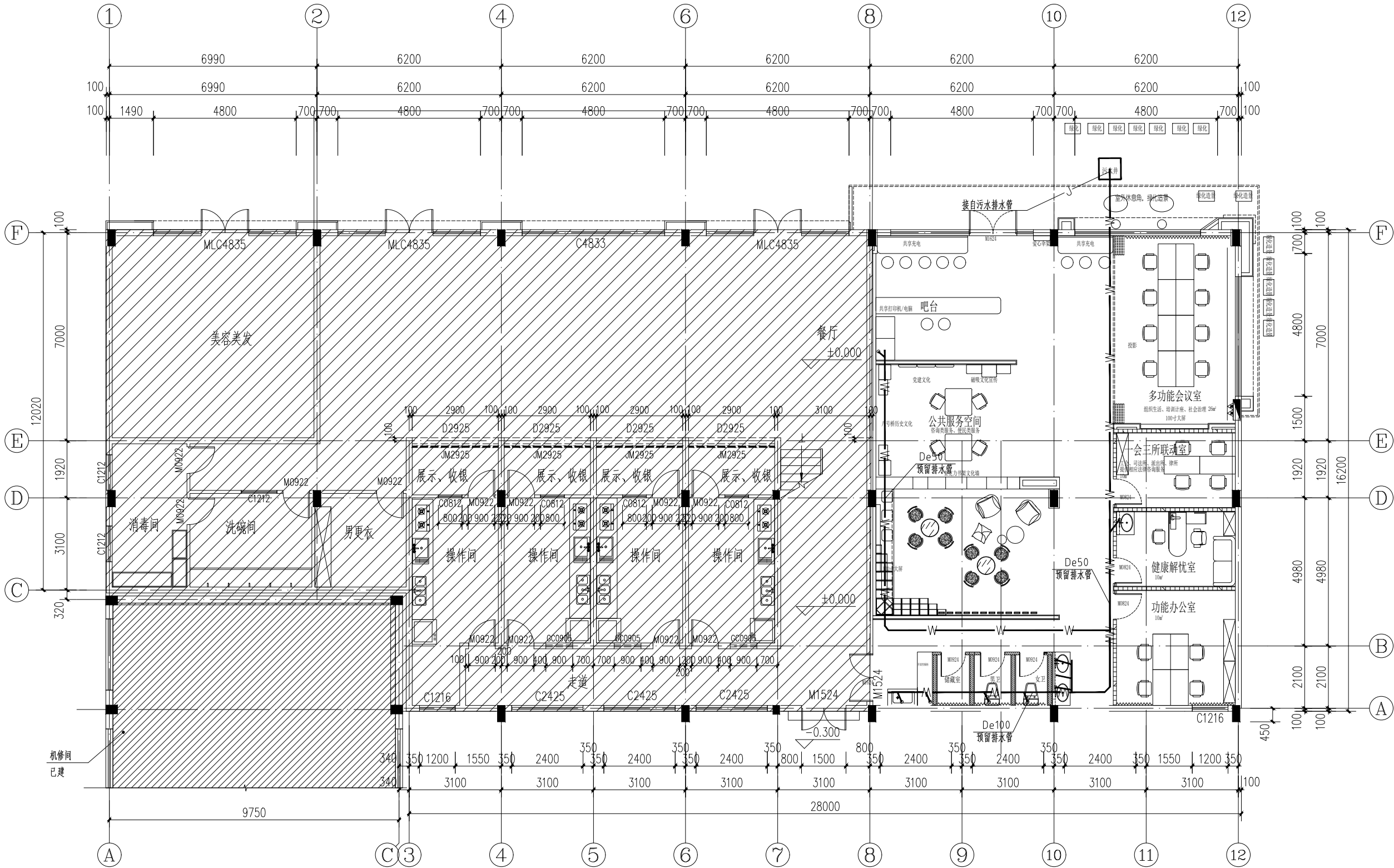
一层排水平面图 1:100
