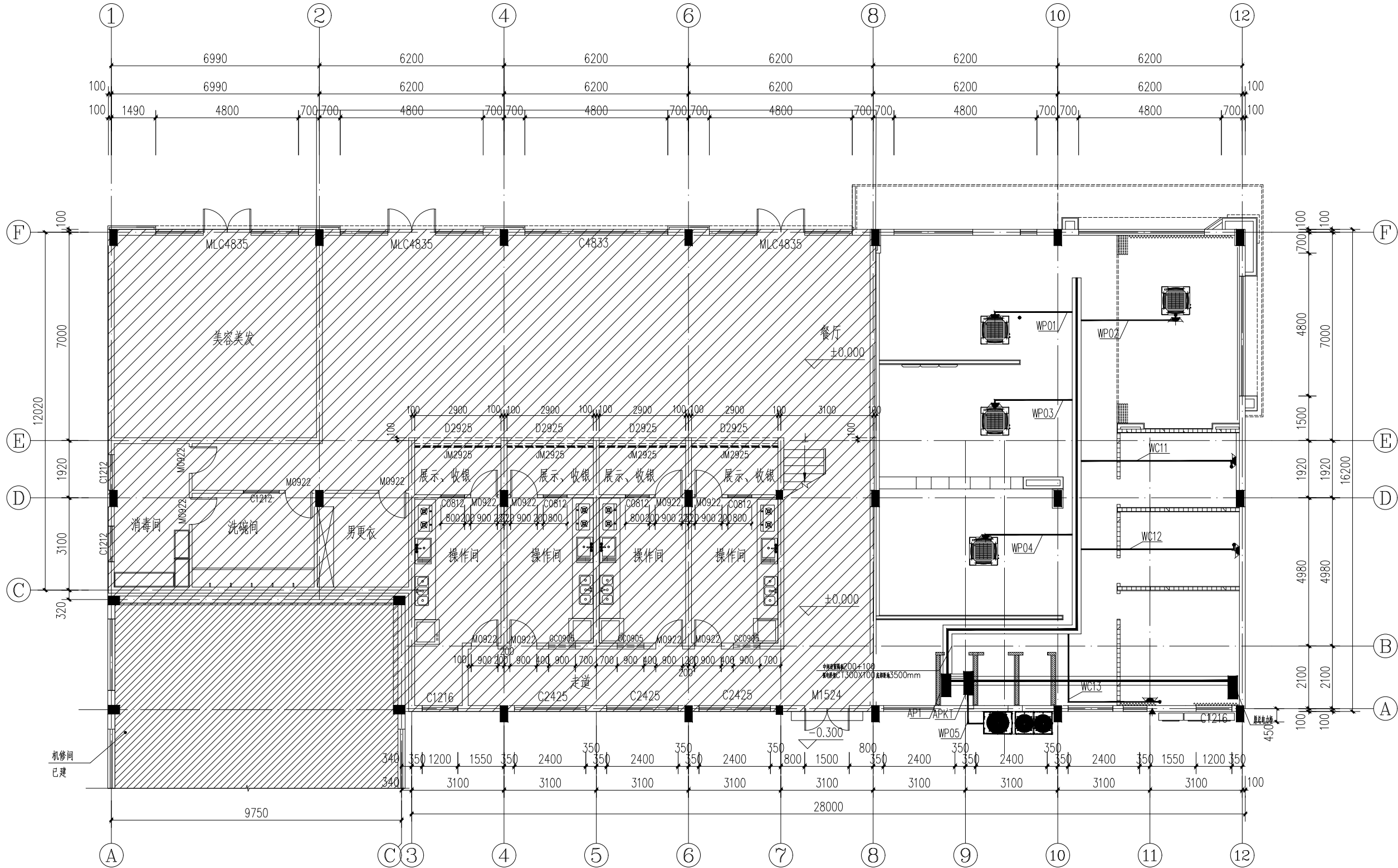
一层空调插座布线图 1:100
