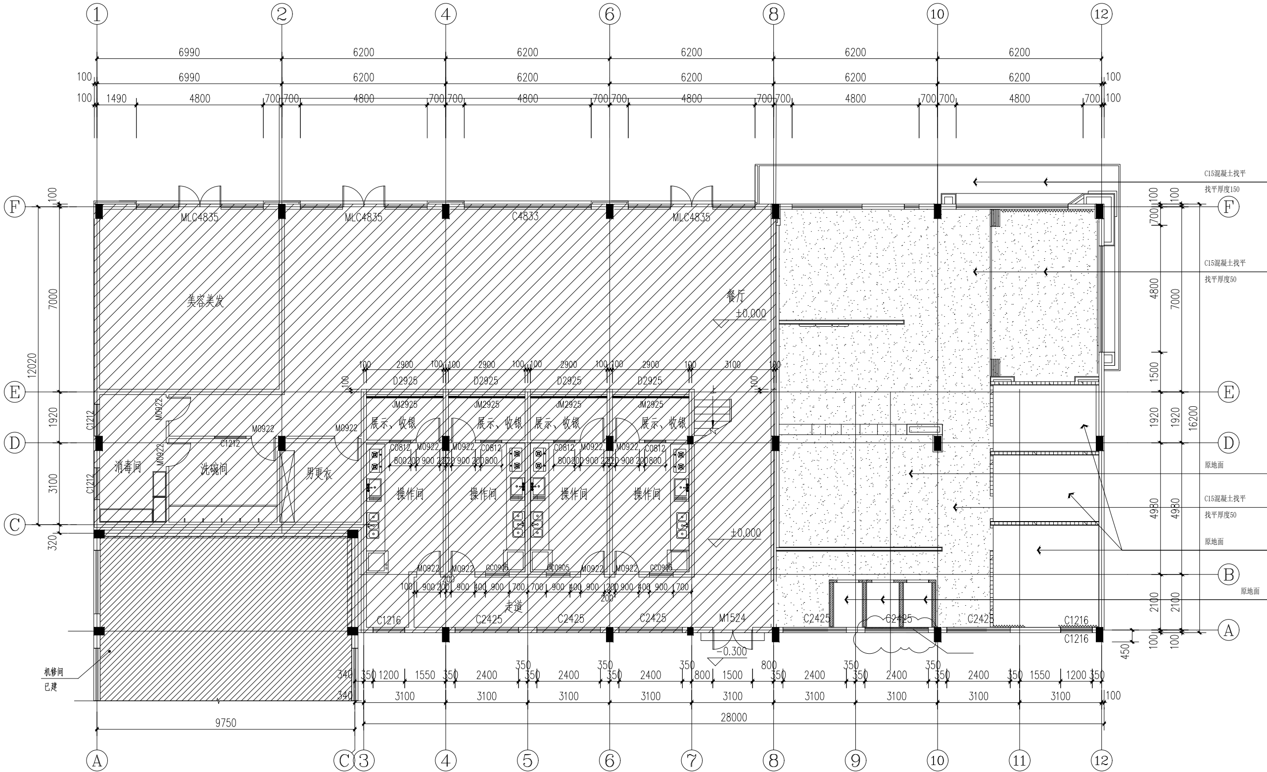
一层地面找坪图 1:100
