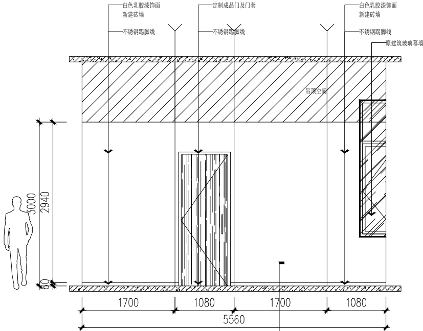
25立面图 比例1:40
