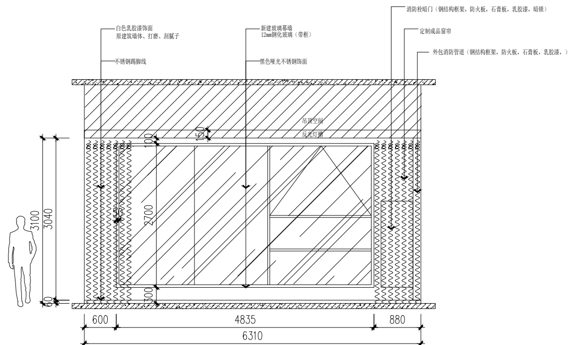
09立面图 比例1:40
