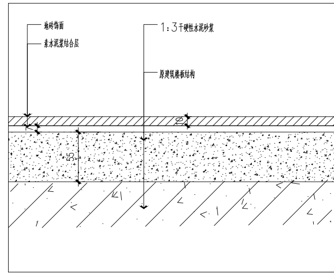
03大样图 比例1:3
