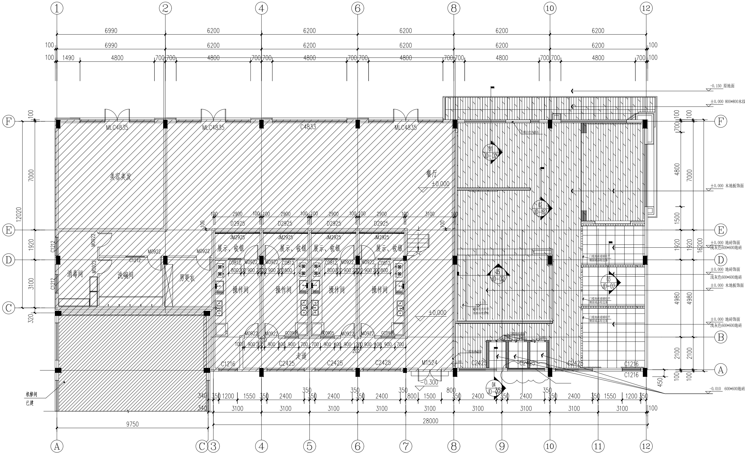
一层地面铺装图 1:100
