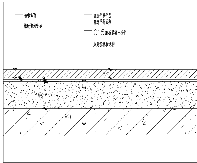
02大样图 比例1:3
