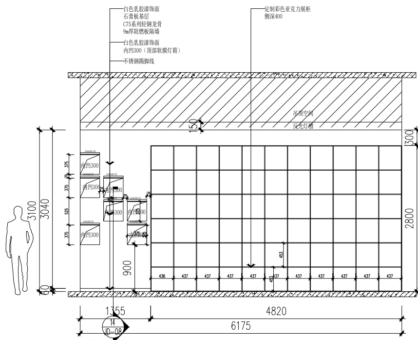
13立面图 比例1:40
