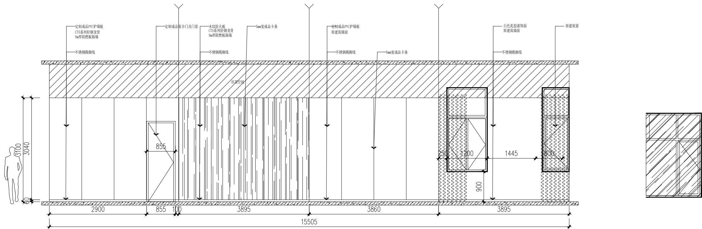
20立面图 比例1:40
