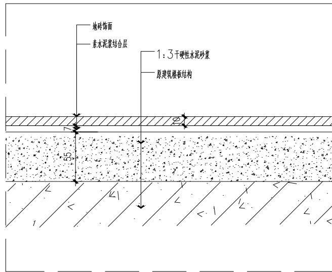
04大样图 比例1:3
