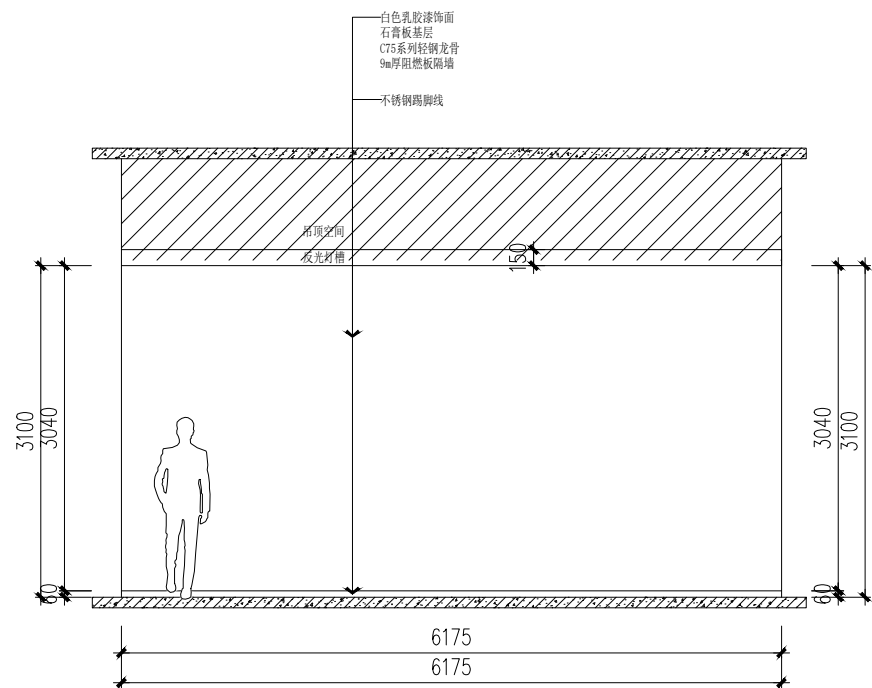
21立面图 比例1:40
