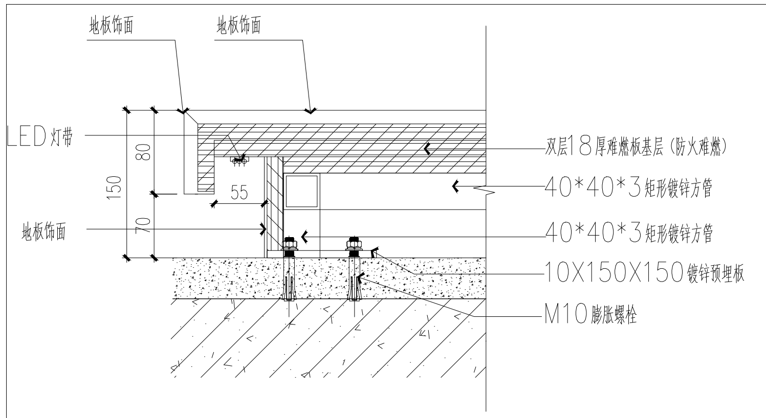
05大样图 比例1:3
