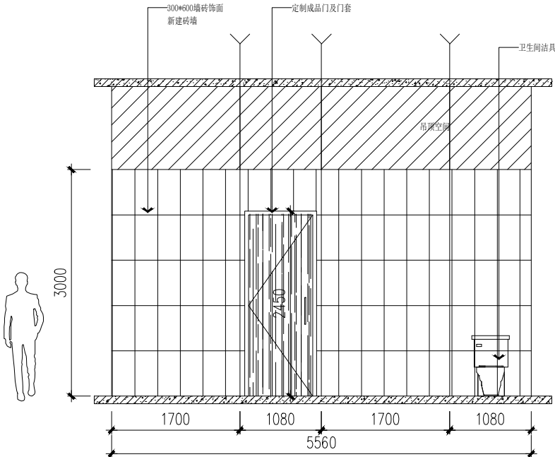
27立面图 比例1:40
