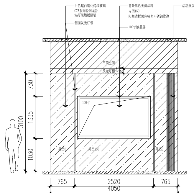
10立面图 比例1:40
