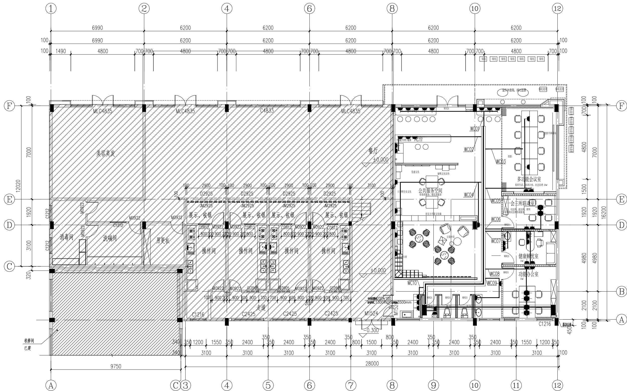
一层插座布线图 1:100
