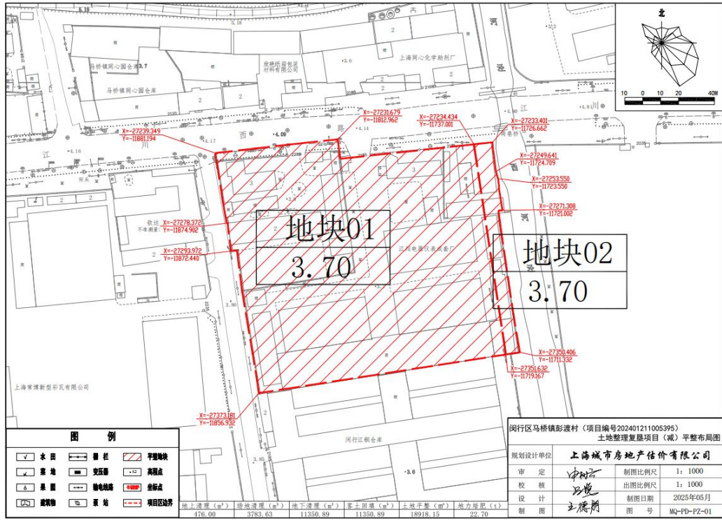
图 3 平整布局
