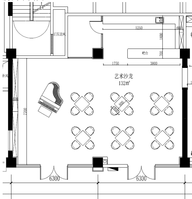
房间平面图
