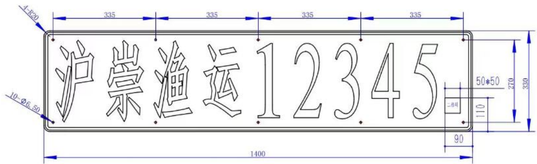
船名牌示意图（单位：mm）
