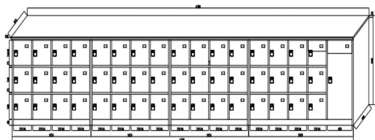
学生储物柜（48小门+1大门）整体示意图：W6300*D420*H1200mm
