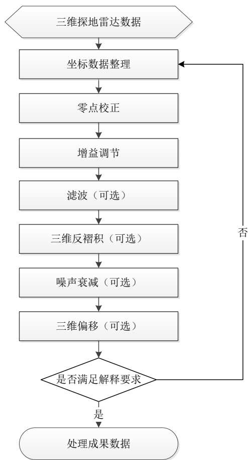
三维探地雷达数据处理流程图
