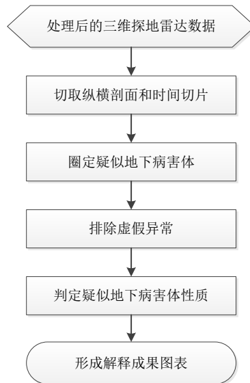
三维探地雷达资料解译流程图
