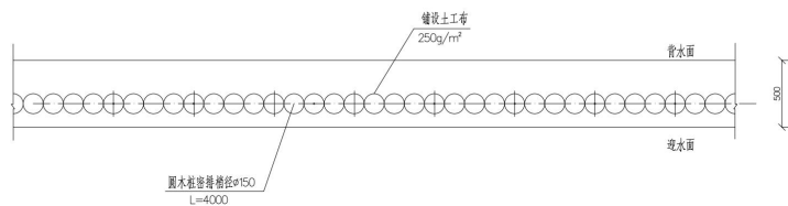
小木桩平面布置图 1:25
