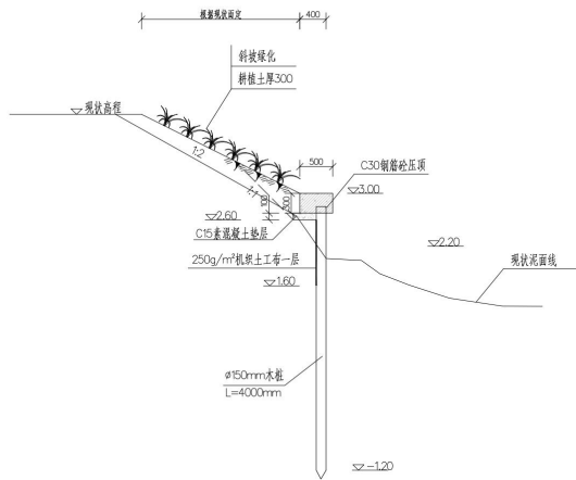
压顶小木桩护岸断面图 1:50
