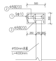
压顶配筋图 1:25
