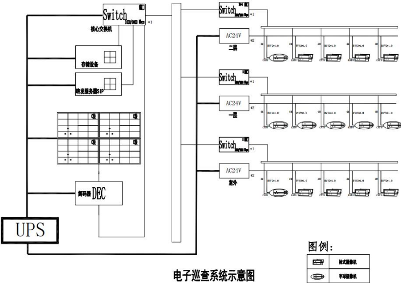
青浦电子巡查网络系统拓扑图：
