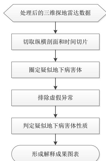
图 3.7.1 三维探地雷达资料解译流程图
