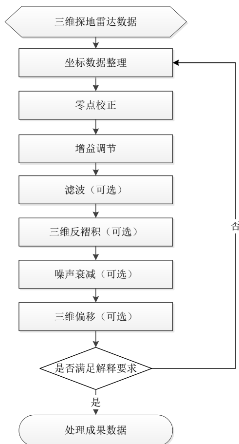
图 3.6.1 三维探地雷达数据处理流程图
