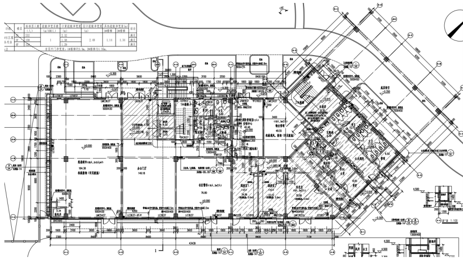
3# 一层平面图
