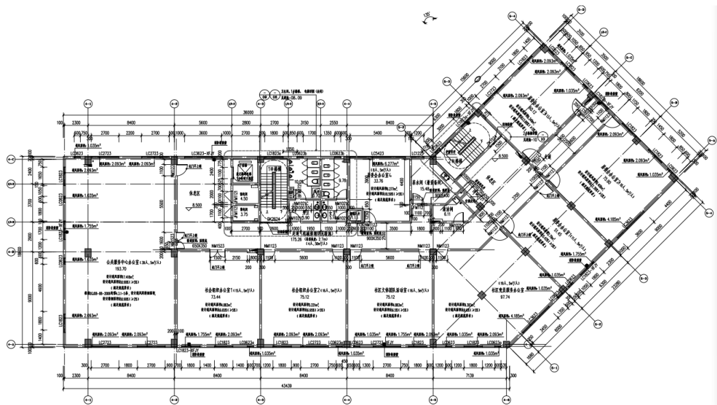
3# 三层平面图
