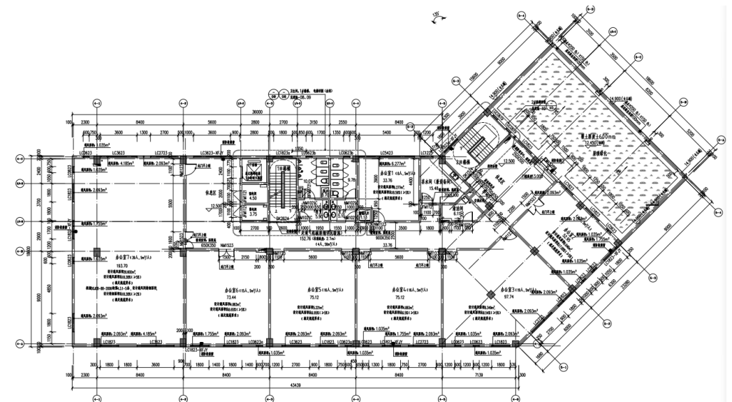
3# 四层平面图
