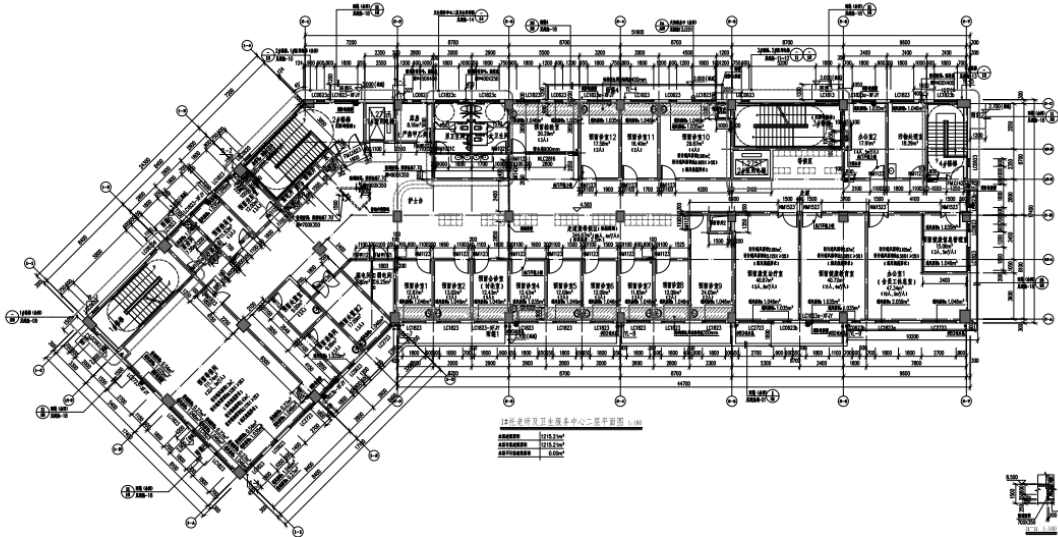
1# 二层平面图
