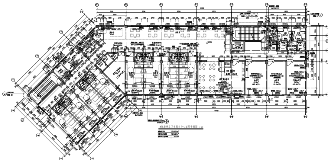
1# 四层平面图
