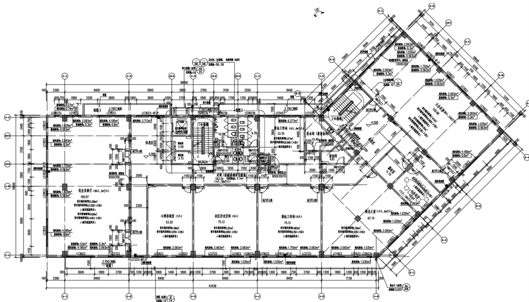
3# 二层平面图
