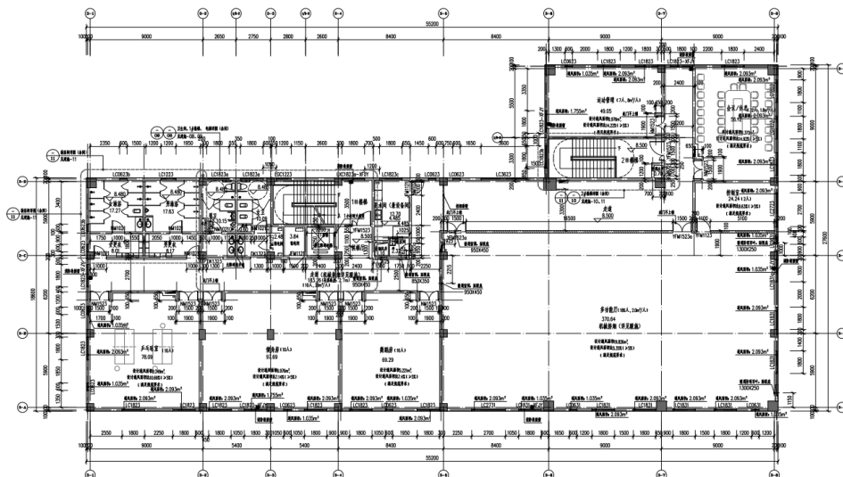
2# 二层平面图
