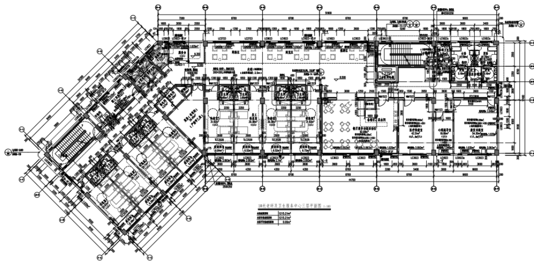
1# 三层平面图
