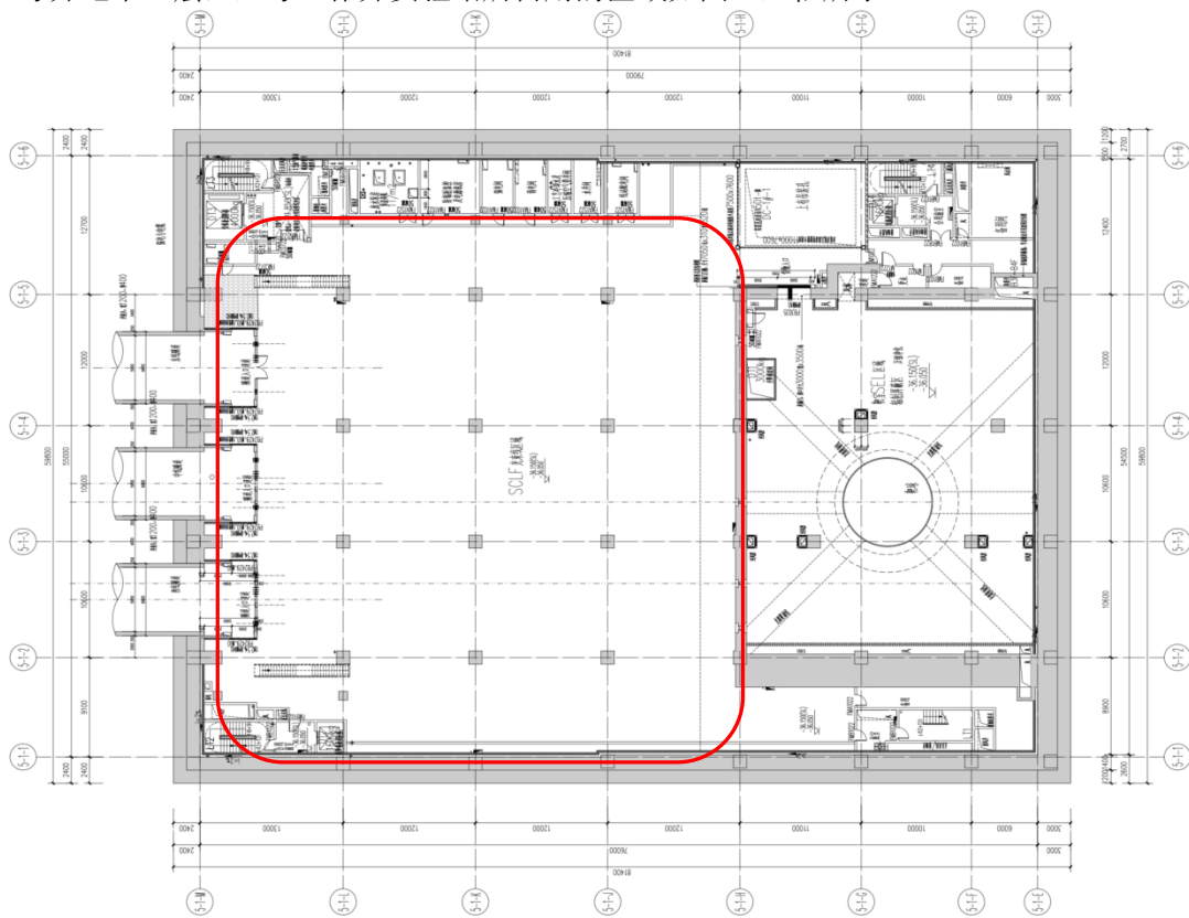
图 2 五号工作井平面图
