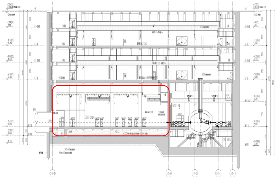
图 1 五号工作井剖面图
