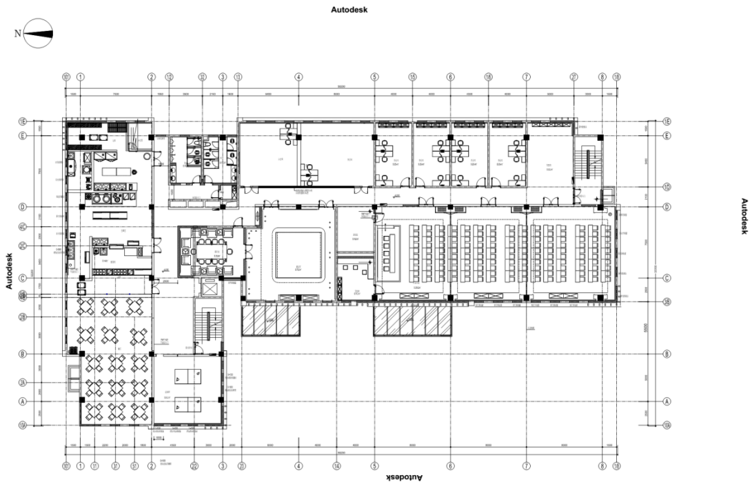
二层平面图
