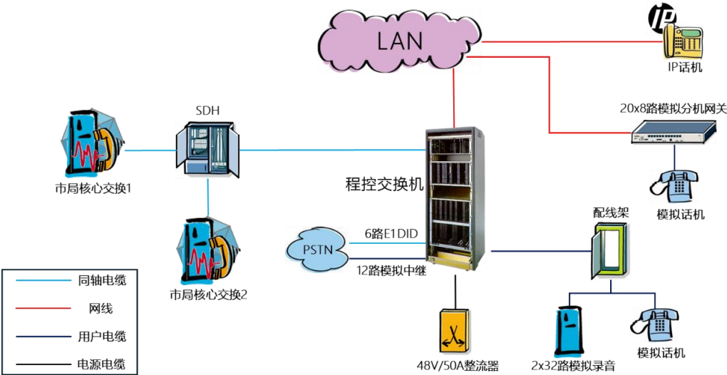
系统拓扑图
