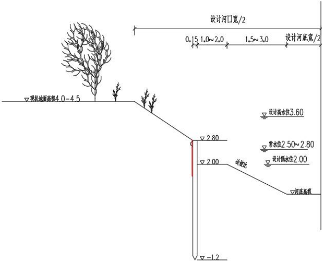
木桩护岸结构图
