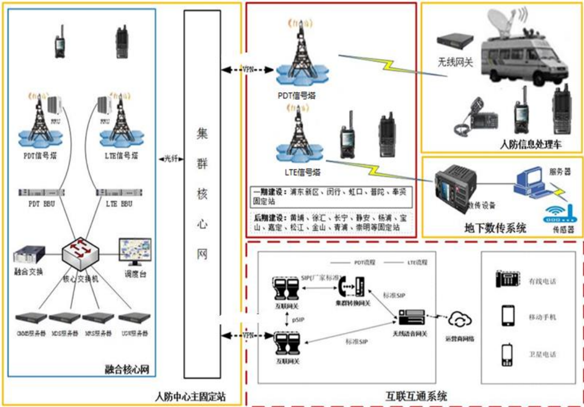
市、区两级系统拓扑图
