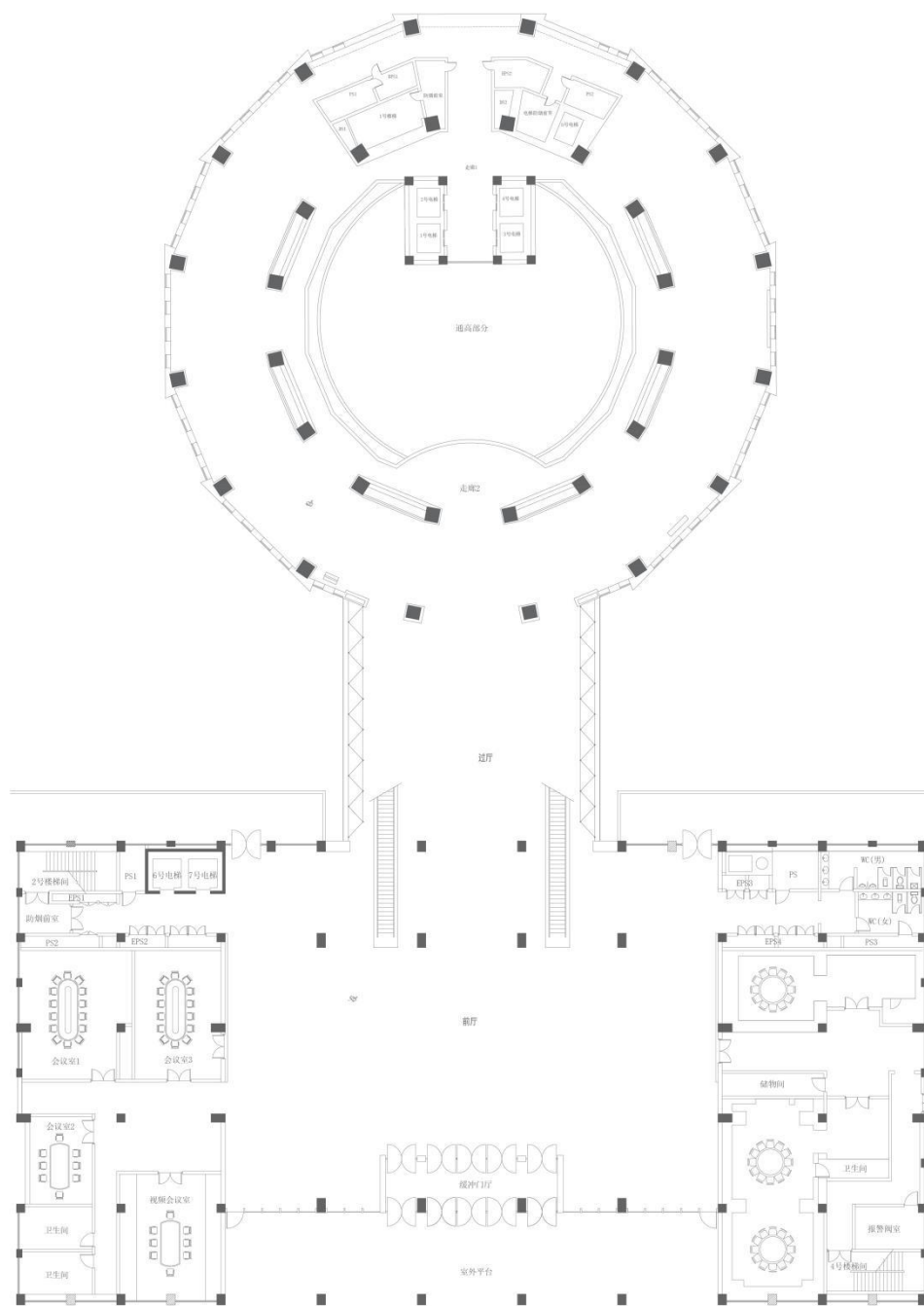
门楼二层平面图
