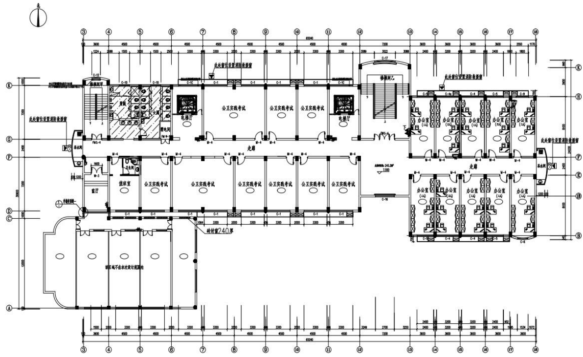
三层平面布置图 1:100 总建筑面积: 1421.00㎡
