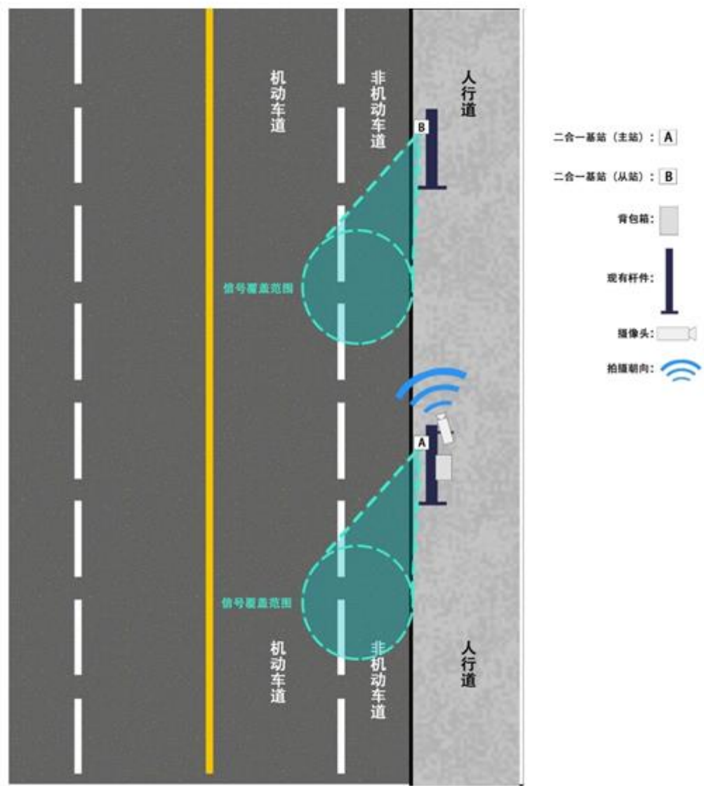
逆向行驶监测安装示意图
