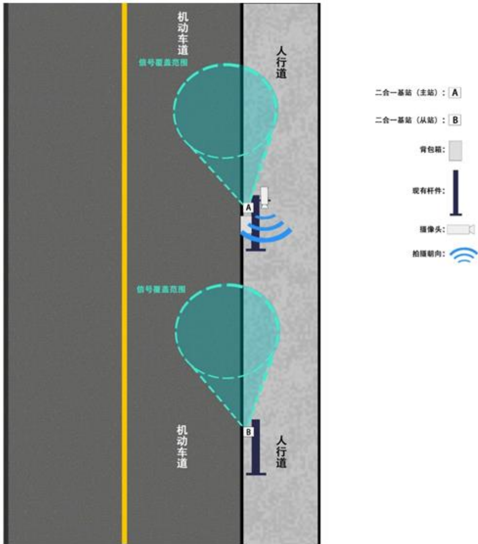
车辆闯禁区监测安装示意图
