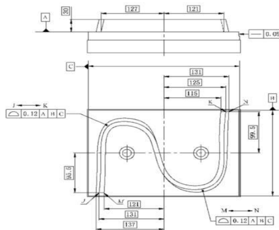
图 10 检验公差图示
