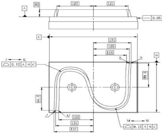
图 10 检验公差图示
