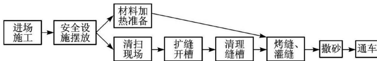
沥青路面修补工艺流程
