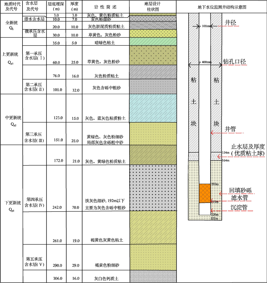
图 1 上海地区典型含水层地下水调查井成井结构示意图
