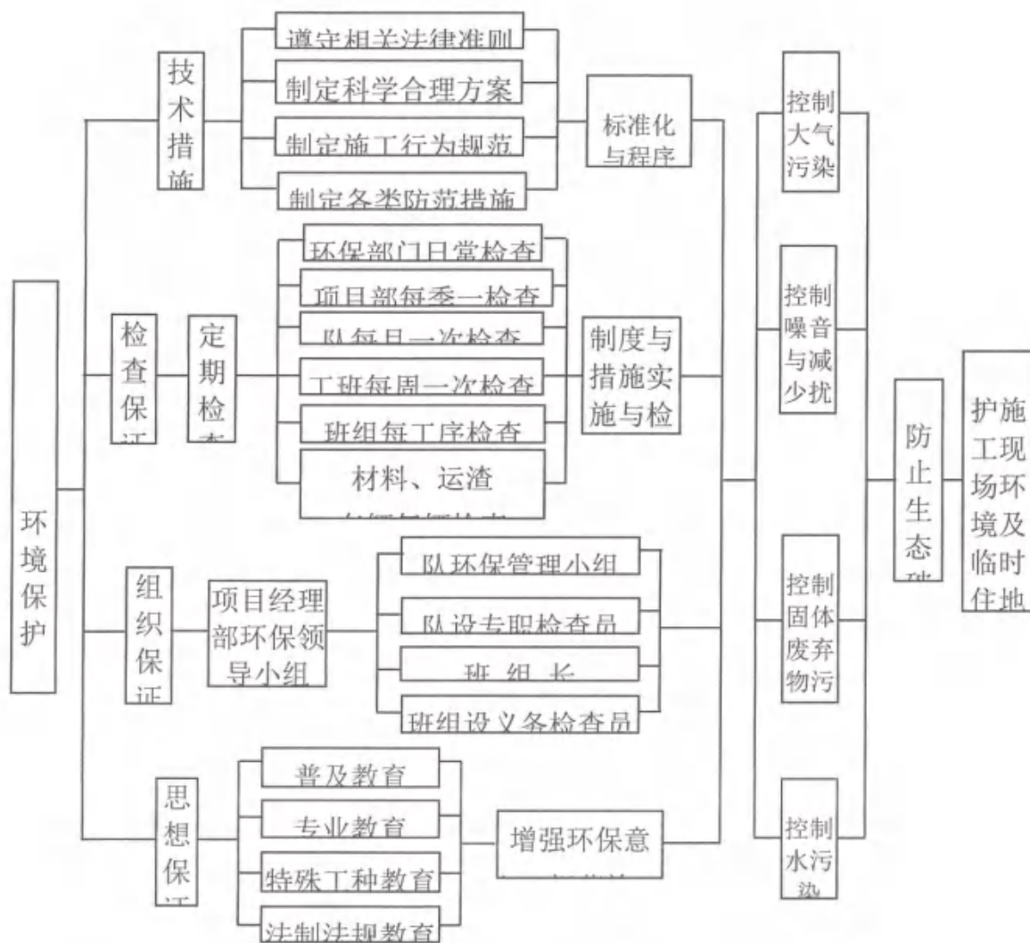
环境保护、水土保持保证管理体系
