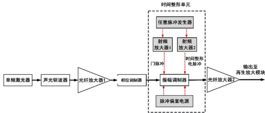
图1.1 纳秒整形前端结构图
