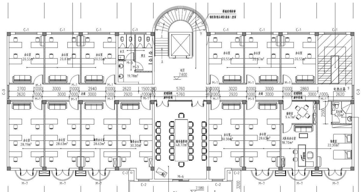
（曲幽路三楼）
