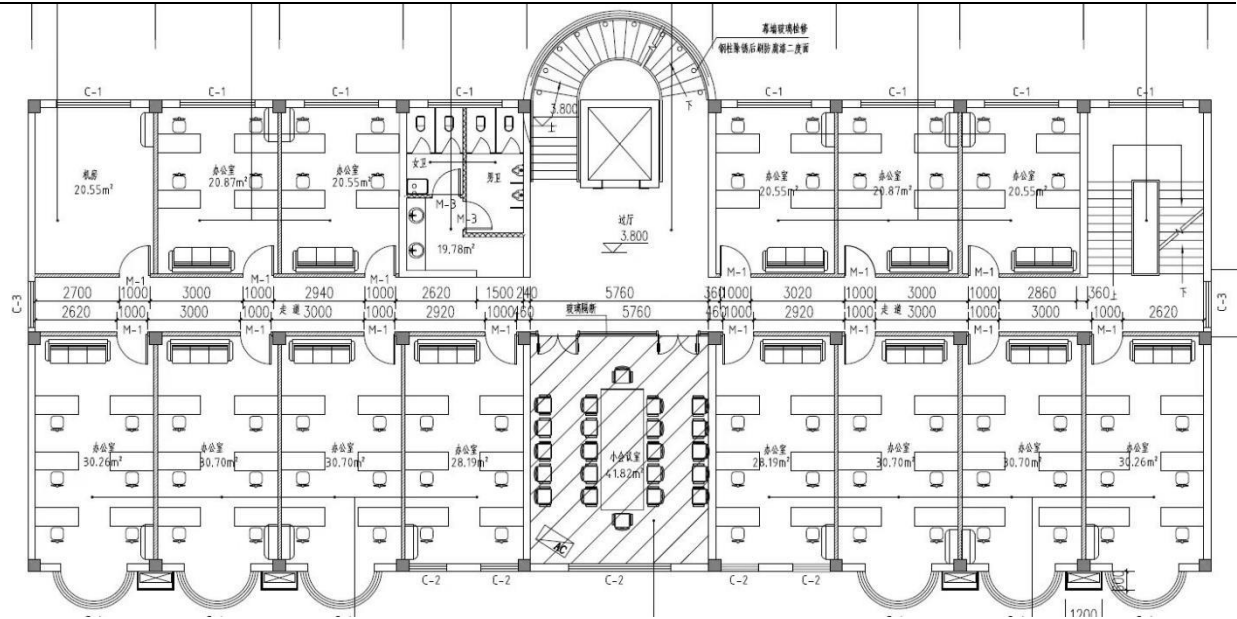
（曲幽路二楼）
