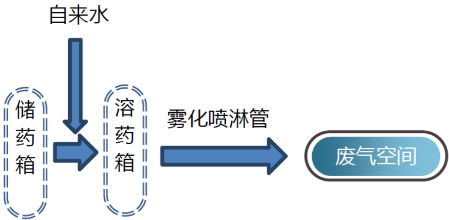
图1-3 植物液喷淋系统工艺流程图
