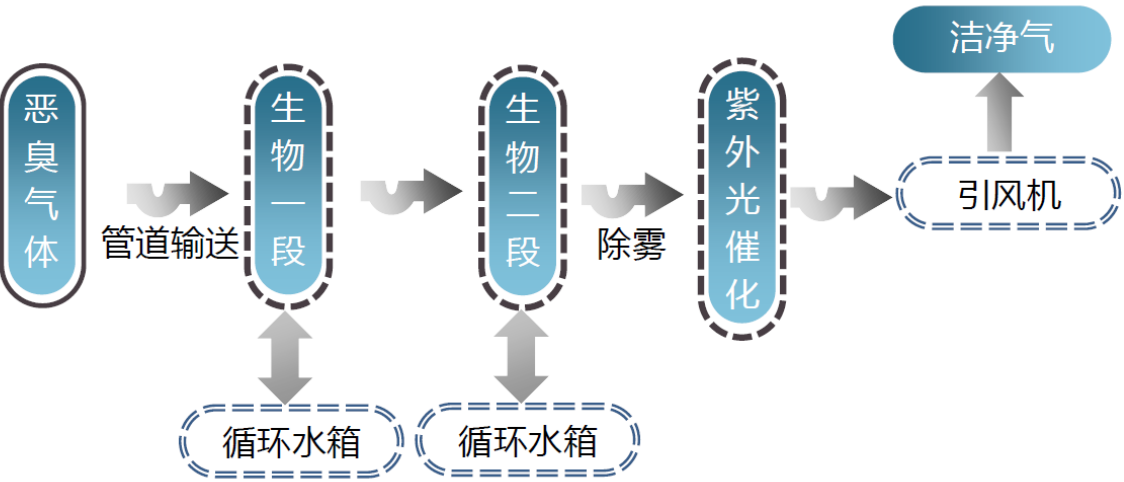
图1-2 集中收集废气处理工艺流程图
