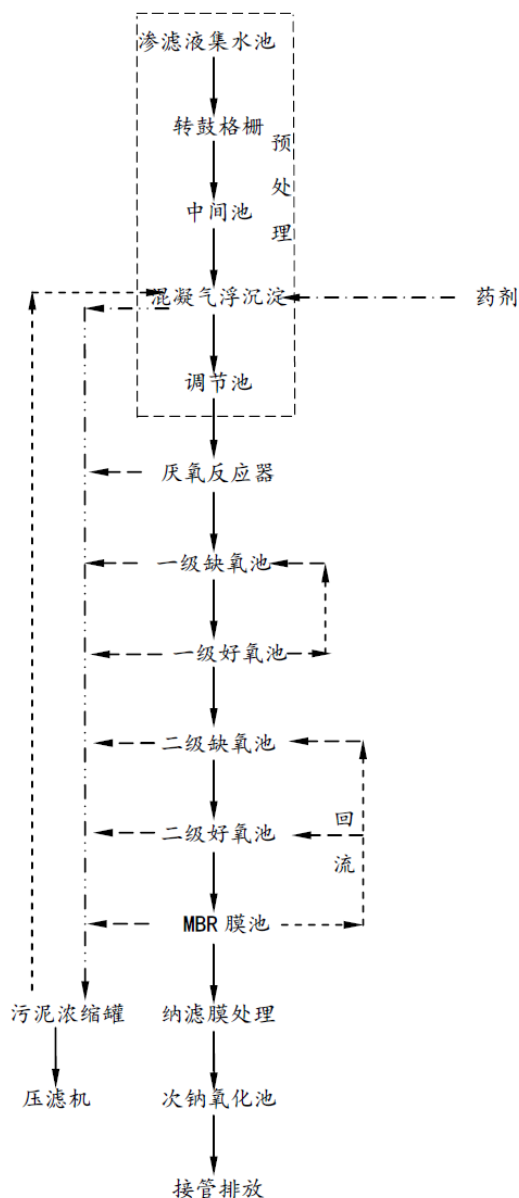
图1-1 渗滤液处理系统工艺流程图
