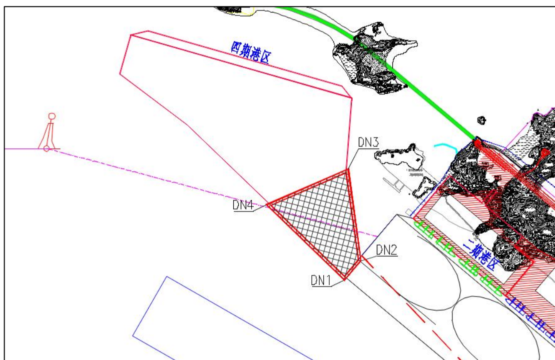
图 4 四期港内水域东南角测量范围示意图
