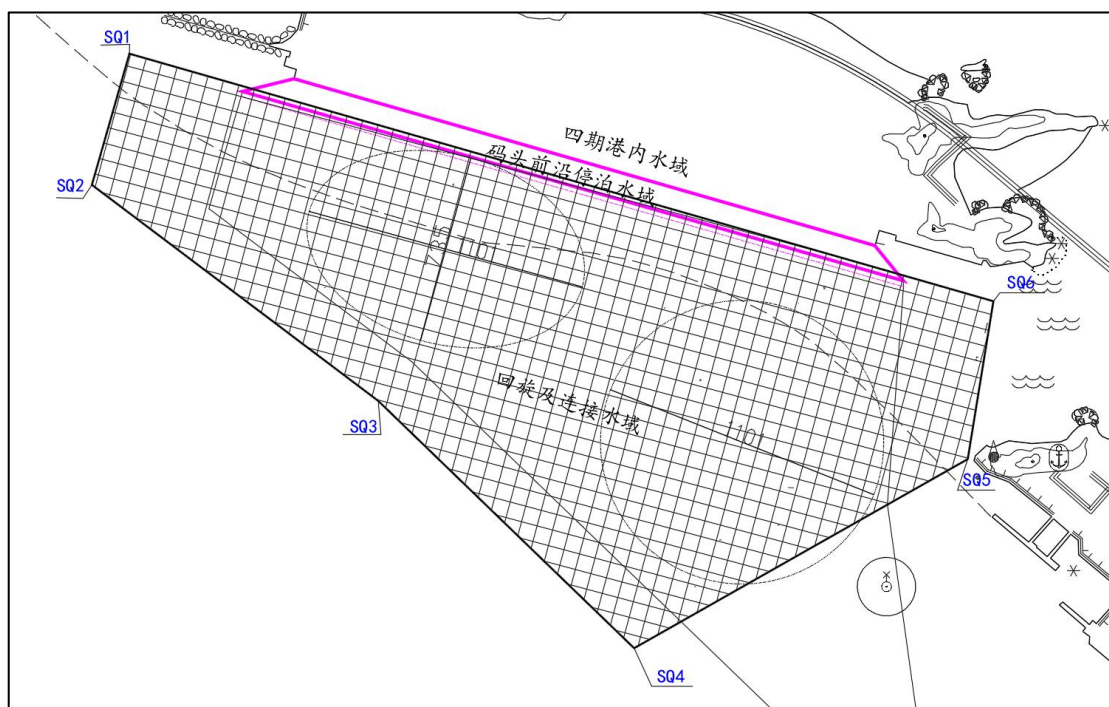
图 5 四期港内水域东南角以外水域测量范围示意图
