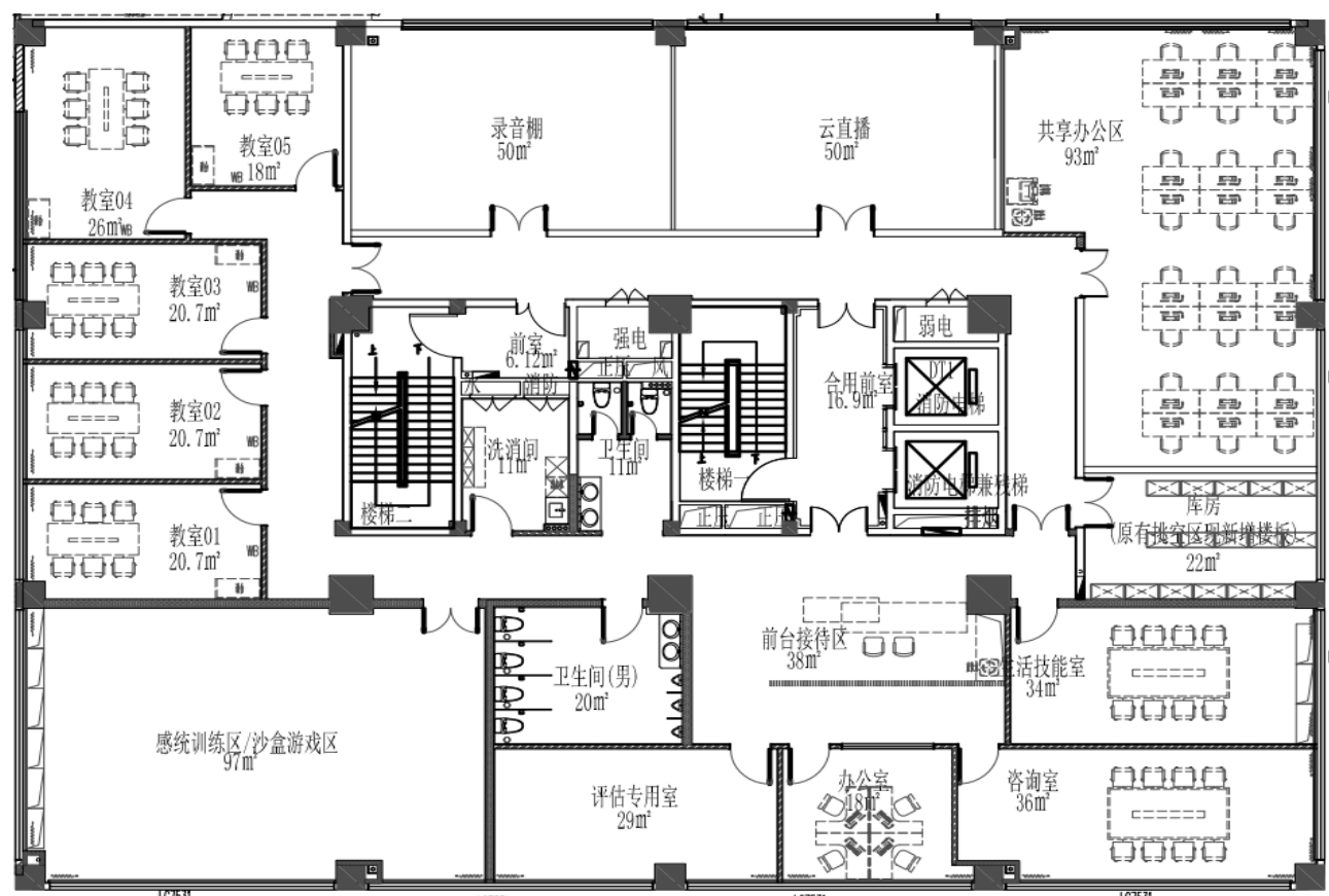
B 区塔楼二层平面图
