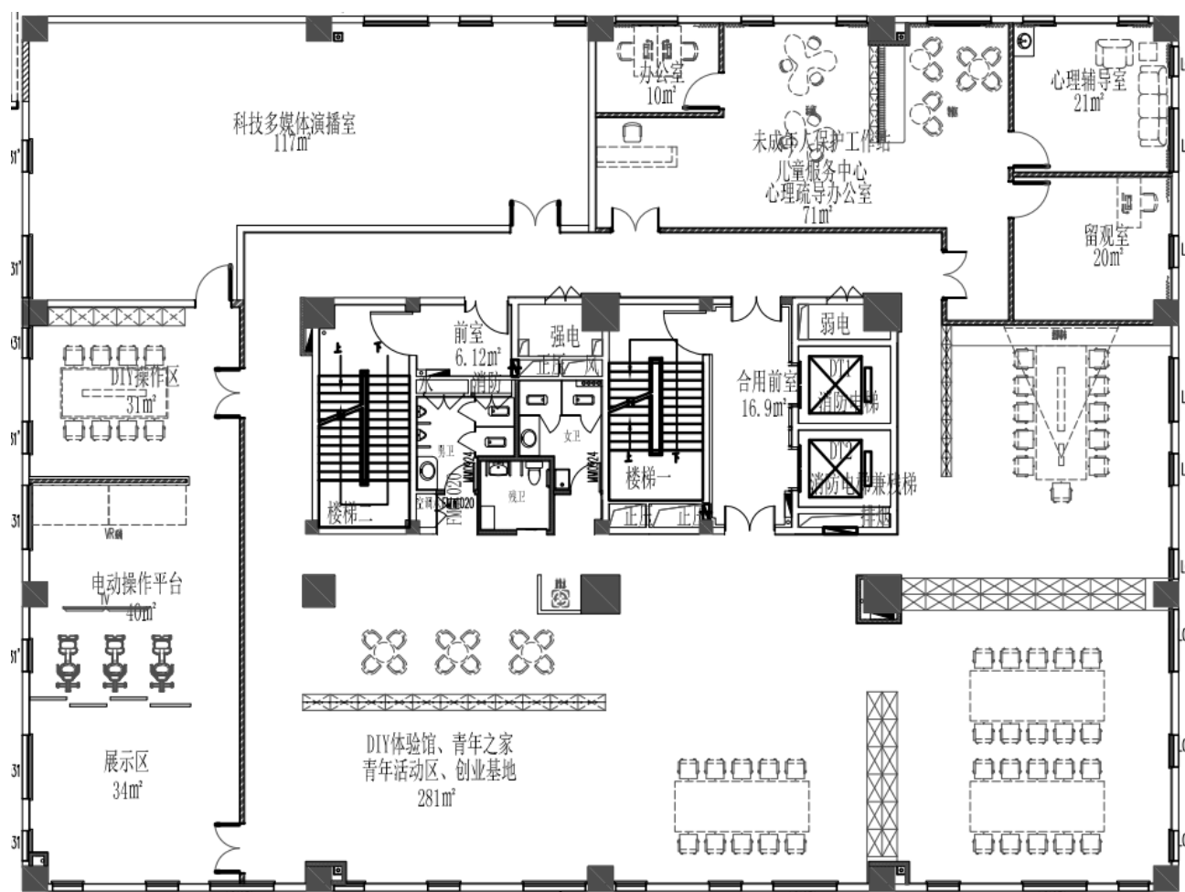
B 区塔楼四层平面图
