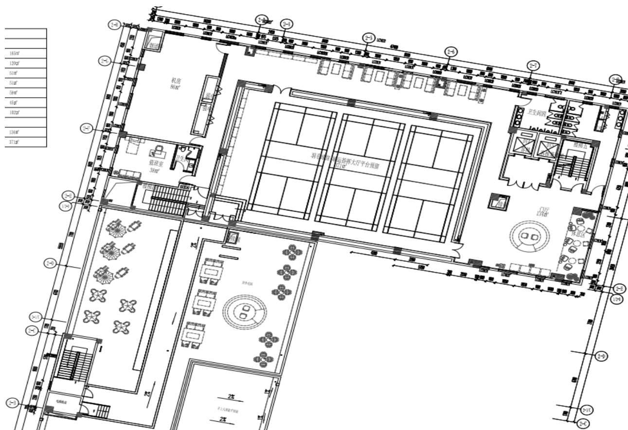
B 区裙楼五层平面图
