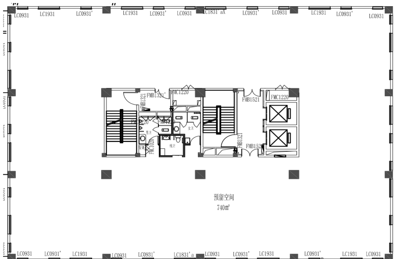
B 区塔楼八层平面图
