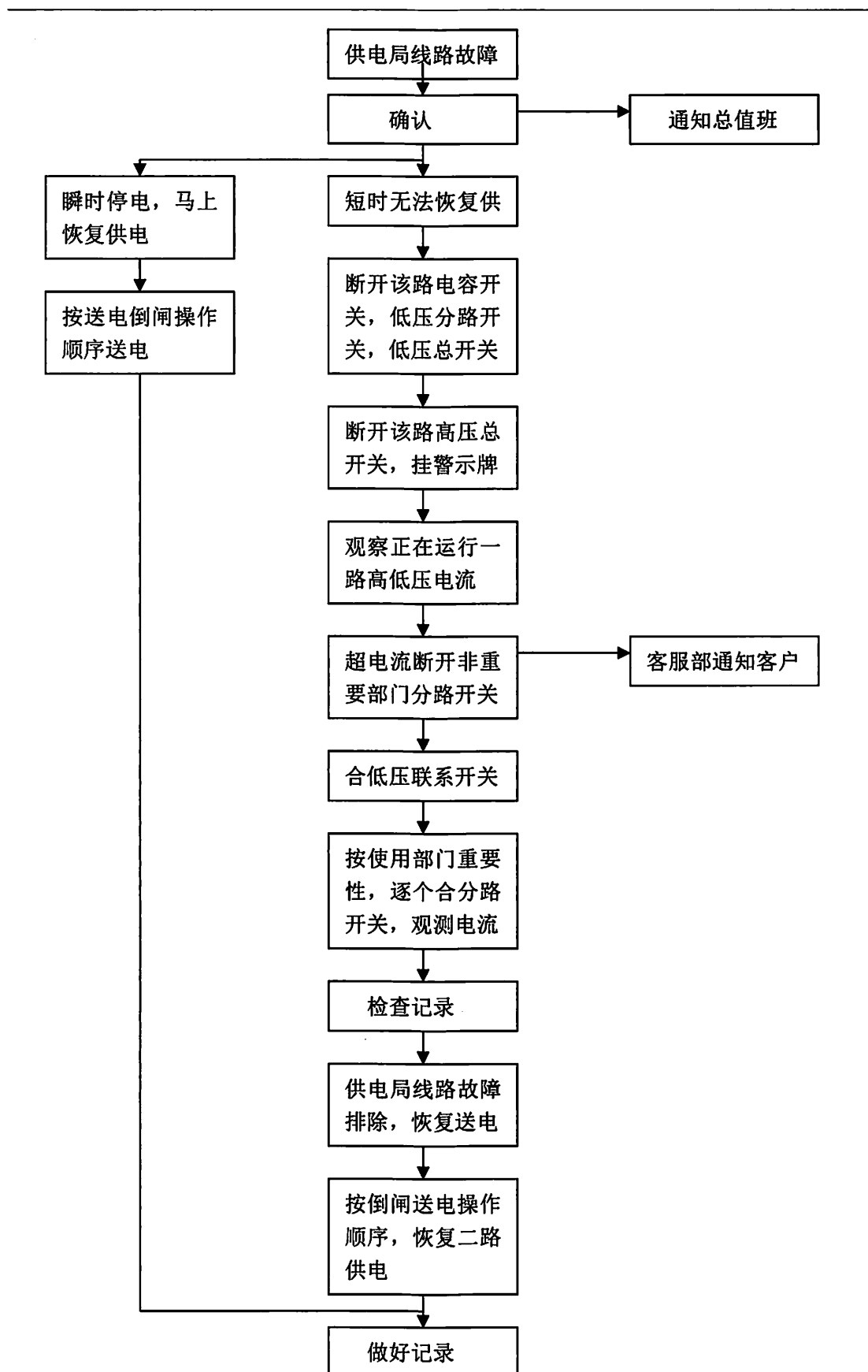
信息数码港外线突发停电应急流程图
