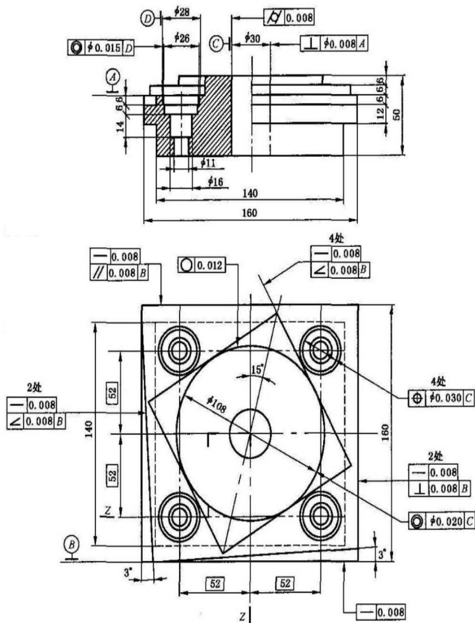
图 2 小规格轮廓加工试件（材质为 304 不锈钢）
