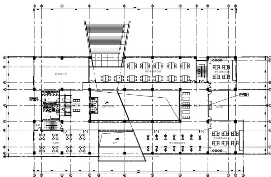
三层平面图
