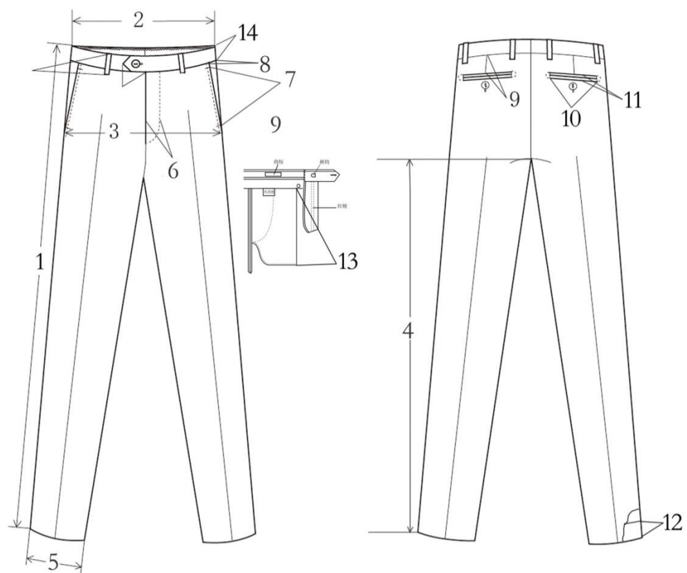
图示 7 男款审判服夏裤成品规格尺寸测量图
