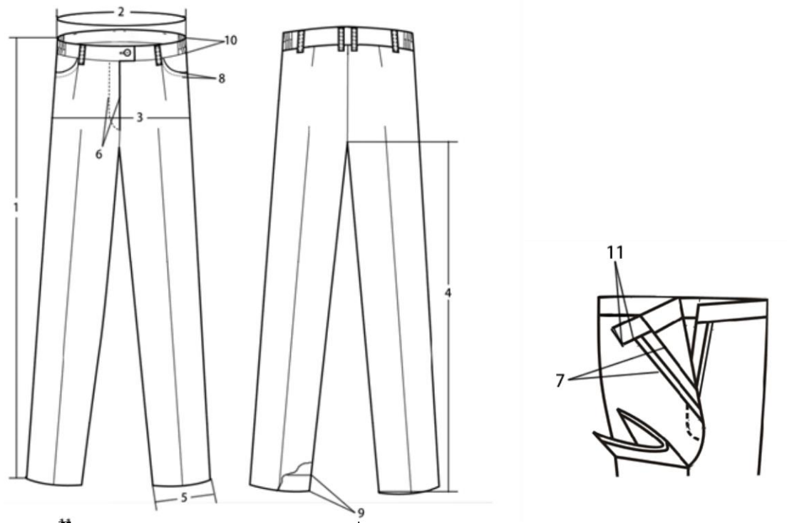
图示 16 女款审判服夏裤成品规格尺寸测量图
