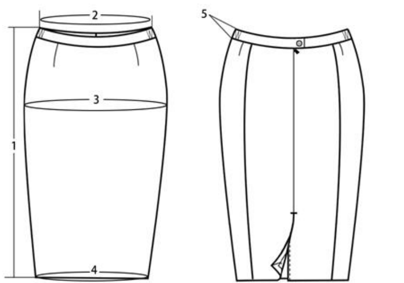
图示 17 女款审判服夏服裙成品规格尺寸测量图
