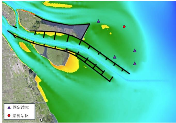
图 2. 拟开展的横沙浅滩水动力泥沙数据采集的点位分布图
