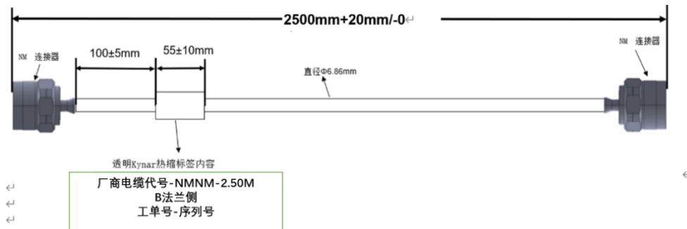
图 2 电缆 2
