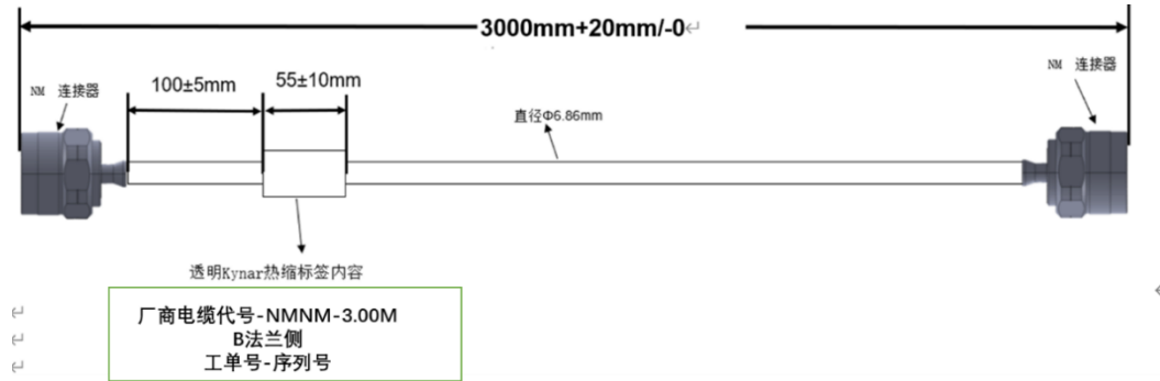
图 3 电缆 3
