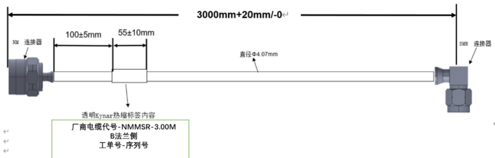
图 1 电缆 1
