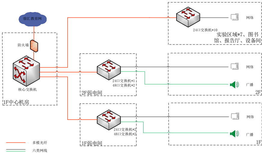
设备网络拓扑图:
