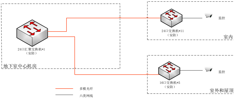
设备网络拓扑图:
