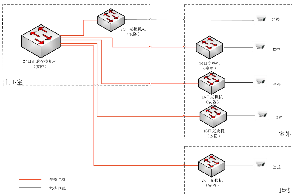
安防网网络拓扑图:
