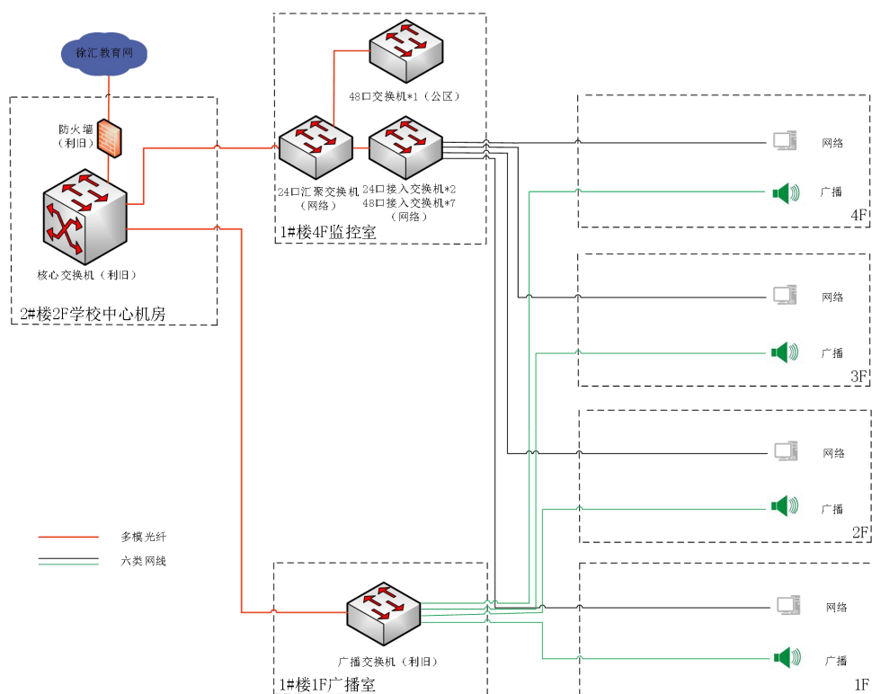
安防网网络拓扑图:
