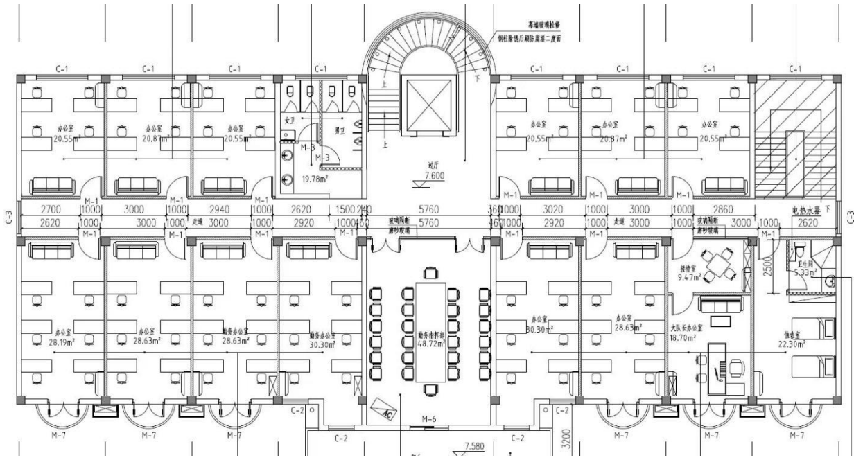
（曲幽路三楼）
