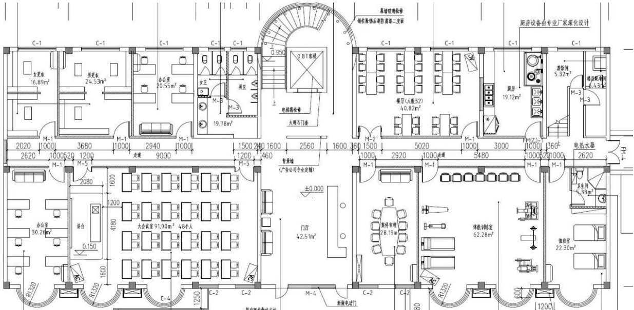
（曲幽路一楼）
