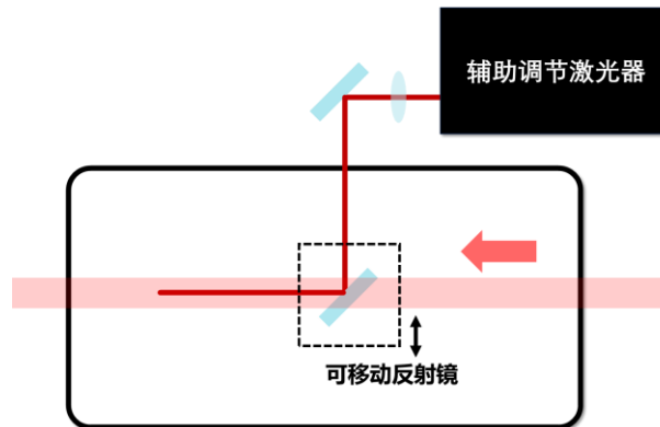
图1.2 辅助调试光源系统光路示意图
